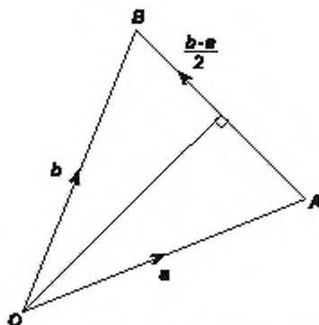
Рисунок 2 — Угол между двумя векторами
