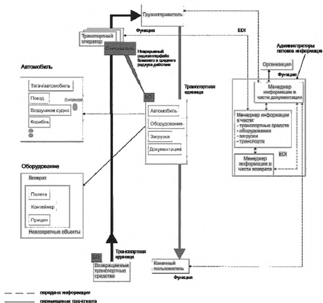
Рисунок 2 — Концептуальный вид системы AVI/AEI
