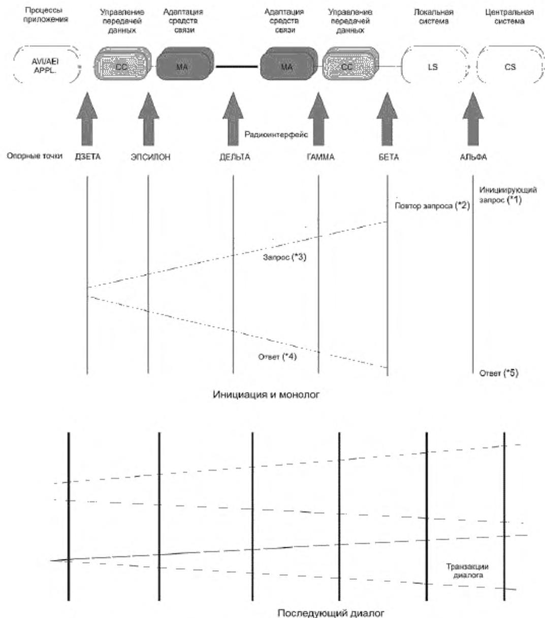
Рисунок 10 — Диаграмма взаимодействия объекта для обобщенной системы AVI/AEI
