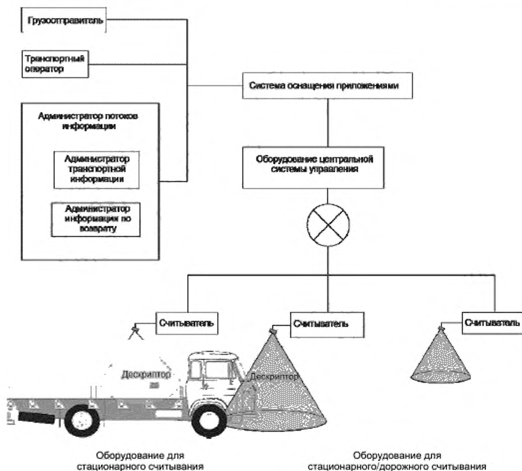
Рисунок 7с — Физическая архитектура
