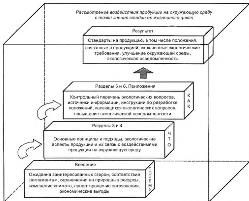
Рисунок 1 — Пошаговый подход для включения экологических аспектов в стандарты на продукцию на основе принципа рассмотрения негативных воздействий продукции на окружающую среду на стадиях жизненного цикла
