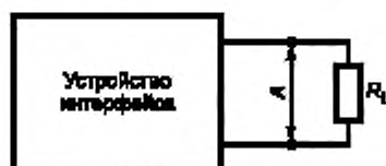
Рисунок 14 — Схема измерения выходных характеристик устройства интерфейса
