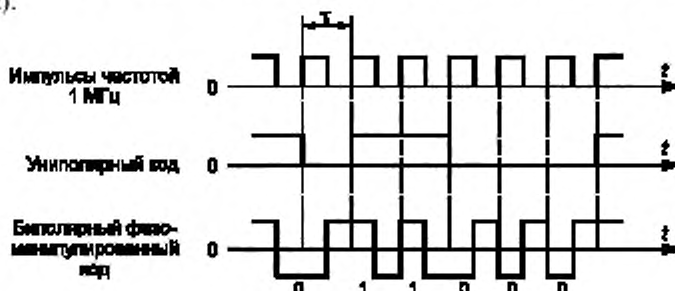
\tau — время передачи одного двоичного разряда
