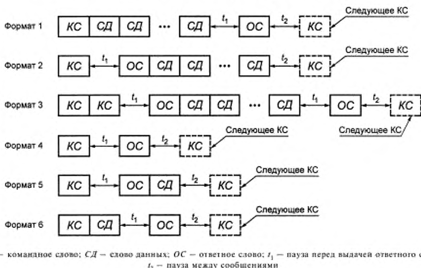
Рисунок 8 — Форматы основных сообщений
