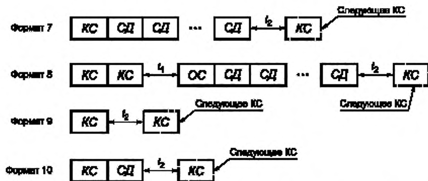
Рисунок 9 — Форматы групповых сообщений
