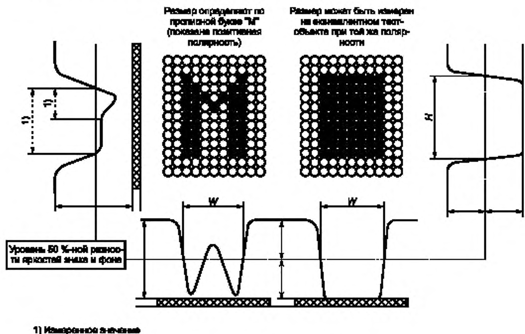
Рисунок 12 — Высота H и ширина W знака
