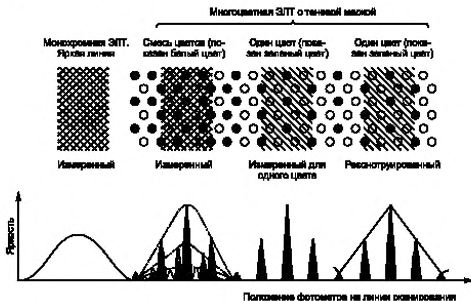
Рисунок 8 — Измеренные и реконструированные профили яркости
