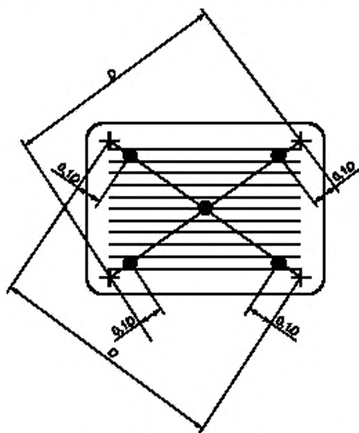
Рисунок 11 — Стандартные места измерений
