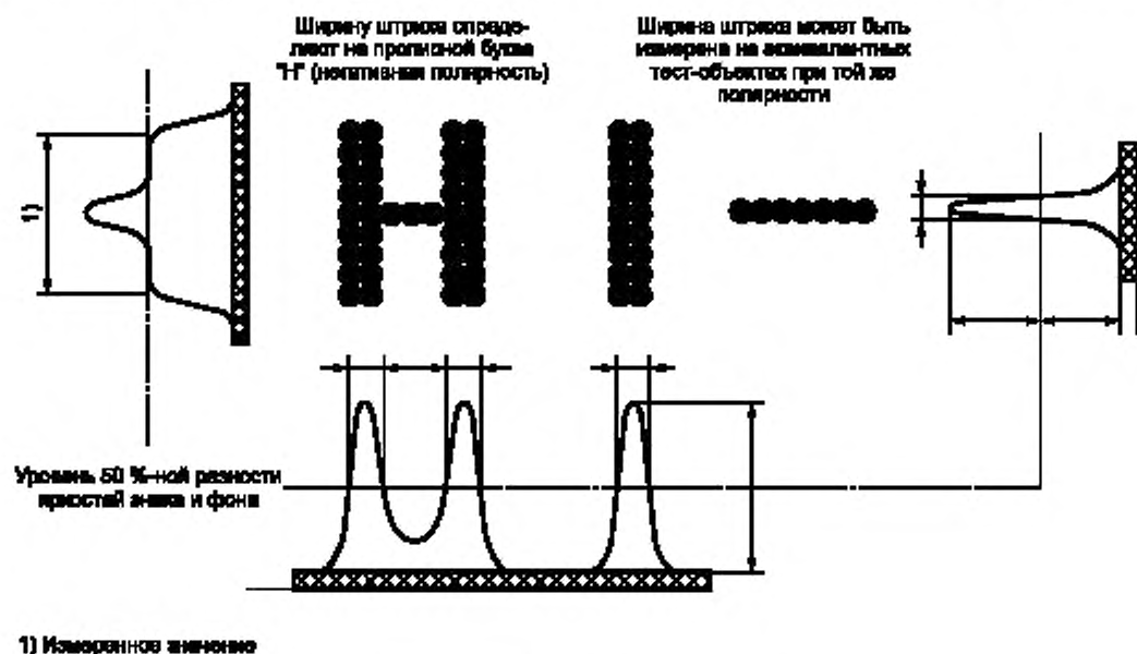
Рисунок 13 — Ширина штриха знака
