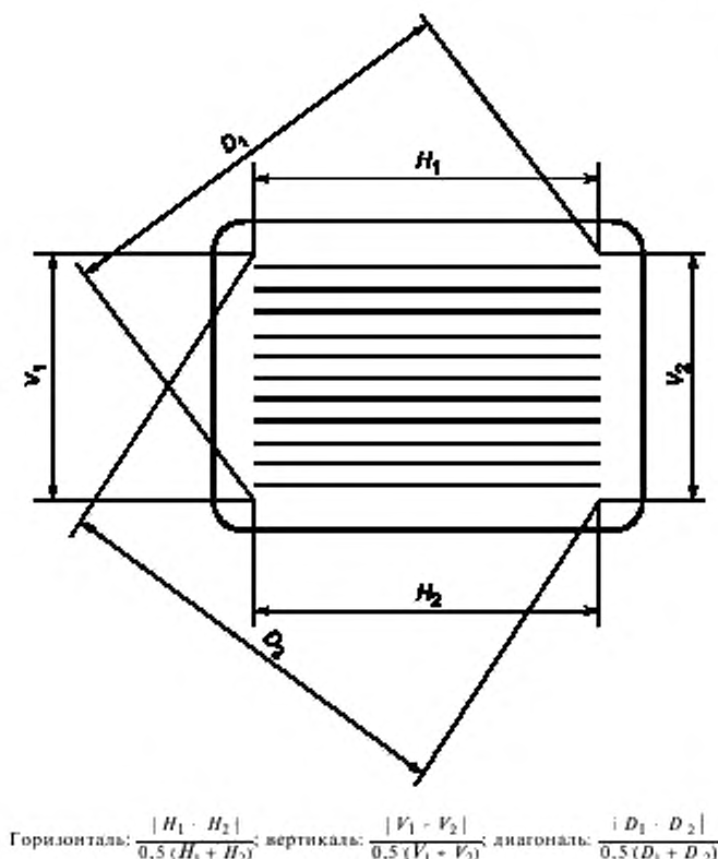
Рисунок 7 — Ортогональность
