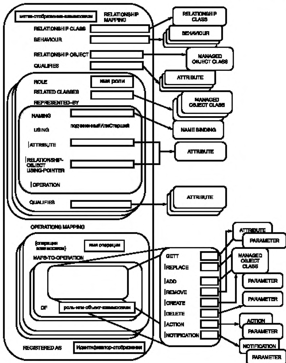
Рисунок Е.2 — Шаблон отображения взаимосвязи
