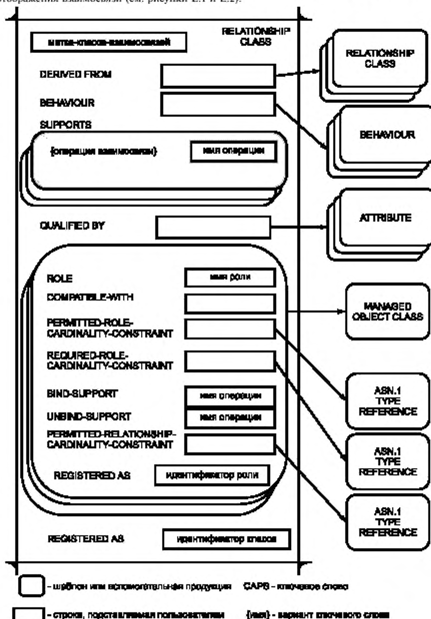
Рисунок Е.1 — Шаблон класса взаимосвязей
