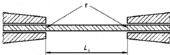
Рисунок 2 — Эффективная длина L_u для испытательных машин с захватом типа блок, применяемых для канатов со ссылочным номером менее 20
