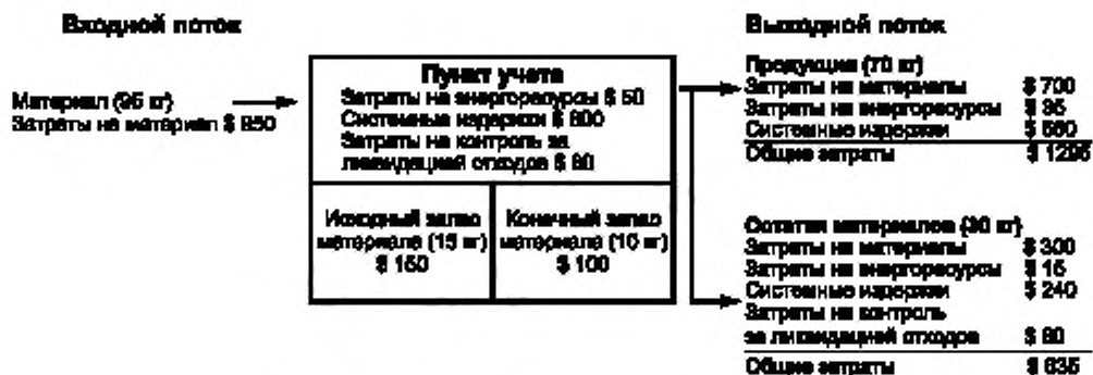
Рисунок 2 — Расчет затрат в пункте учета(QC-пункте)
