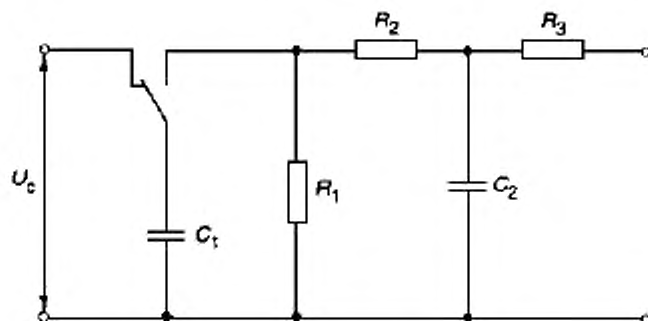
Рисунок N.1 — Схема испытательного генератора импульсов МСЭ-Т
