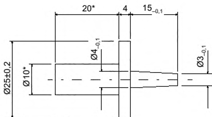
Рисунок 2В — Испытательный штырь
