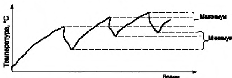
Рисунок В.1 — Определение среднеарифметического значения температуры
