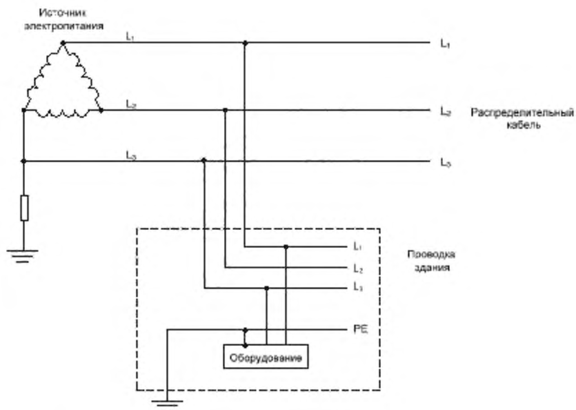
Рисунок V.8 — Пример IT-системы электропитания с тремя фазами
