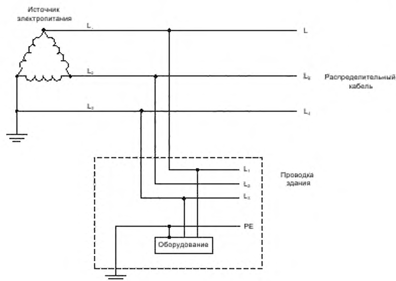
Рисунок V.6 — Пример ТТ-системы электропитания с тремя фазами
