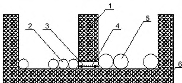
Рисунок F.17 — Компонент, заполненный изоляционным компаундом
