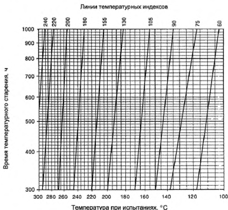
Рисунок 2J — Время теплового старения
