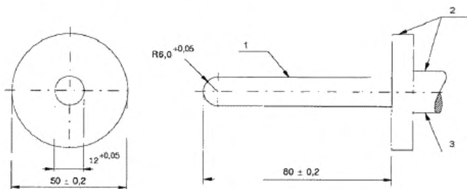
Рисунок 2С — Испытательный шуп
