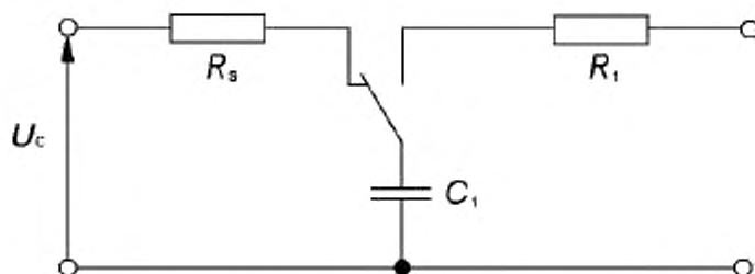
Рисунок N.2 — Схема испытательного генератора импульсов по IEC 60065
