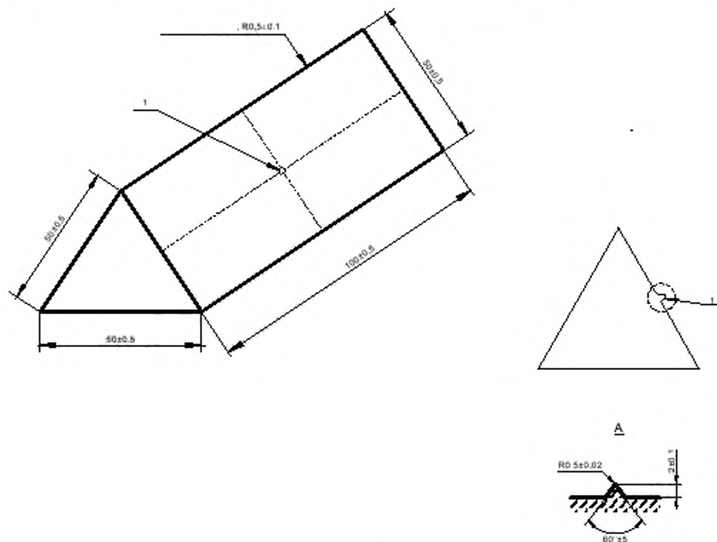
Рисунок АА.1 — Оправка
