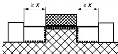
Рисунок F.6 — Нескрепленный стык с широкими канавками
