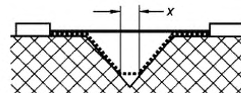
Рисунок F.3 — V-образная канавка
