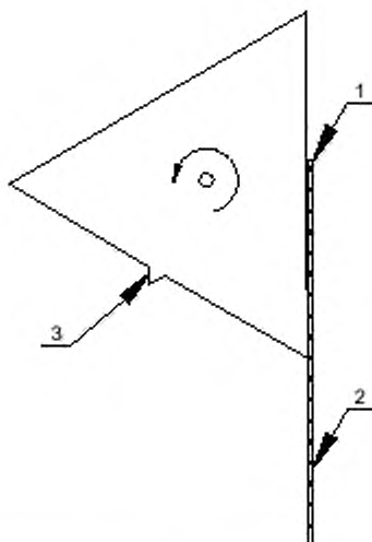
1 — крепежный элемент, 2 — изоляционный материал; 3 — шип
