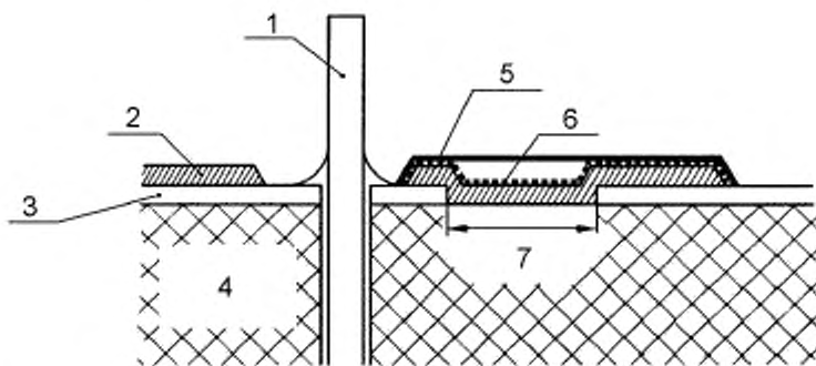
Рисунок F.10 — Покрытие вокруг выводов
