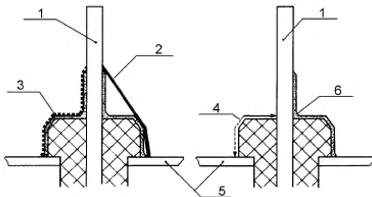
Рисунок F.9 — Широкое углубление
