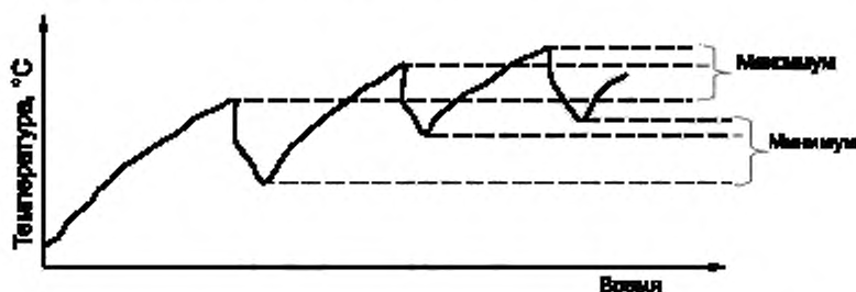
Рисунок С.1 — Определение среднеарифметического значения температуры
