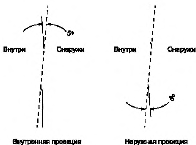
Рисунок 4C — Примеры конструкции жалюзи
