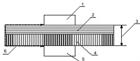
Рисунок F.14 — Сплошной изоляционный материал
