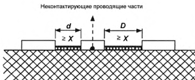
Рисунок F.13 — Интервал, несоединенная проводящая часть
