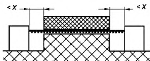
Рисунок F.5 — Нескрепленный стык с узкими канавками
