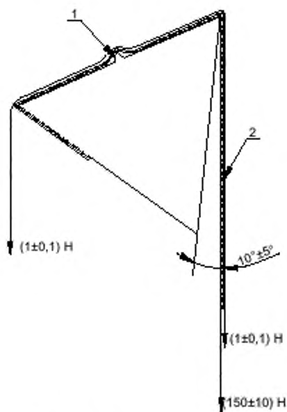
1 — шип; 2 — металлическая фольга
