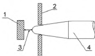
Рисунок 2С — Испытательный шуп
