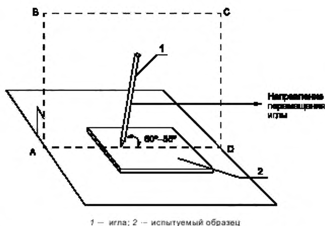
Рисунок 2К — Испытание покрывающего слоя на износостойкость
