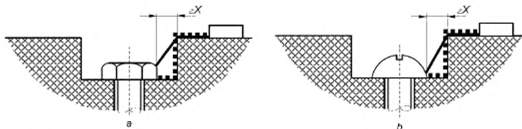
Рисунок F.9 — Широкое углубление
