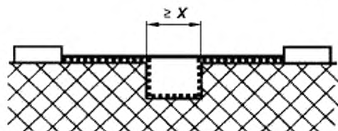
Рисунок F.2 — Широкая канавка
