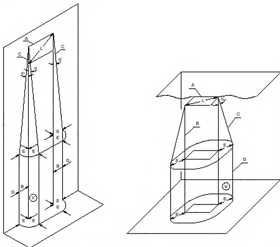
A — отверстие в кожухе; B — вертикальная проекция внешних кромок отверстия; C — наклонные линии под углом 5^\circ к кромкам бокового отверстия, расположенные на расстоянии E от B; D — линия, проведенная вертикально вниз в плоскости боковой стенки кожуха; E — проекция отверстия (не должна быть более L); L — максимальный размер бокового отверстия кожуха, V — объем, в котором не должны быть расположены оголенные части, находящиеся под опасным напряжением или части, представляющие собой энергетическую опасность
