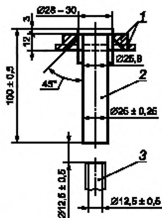
1 — держатель; 2 — образец; 3 — сопло
