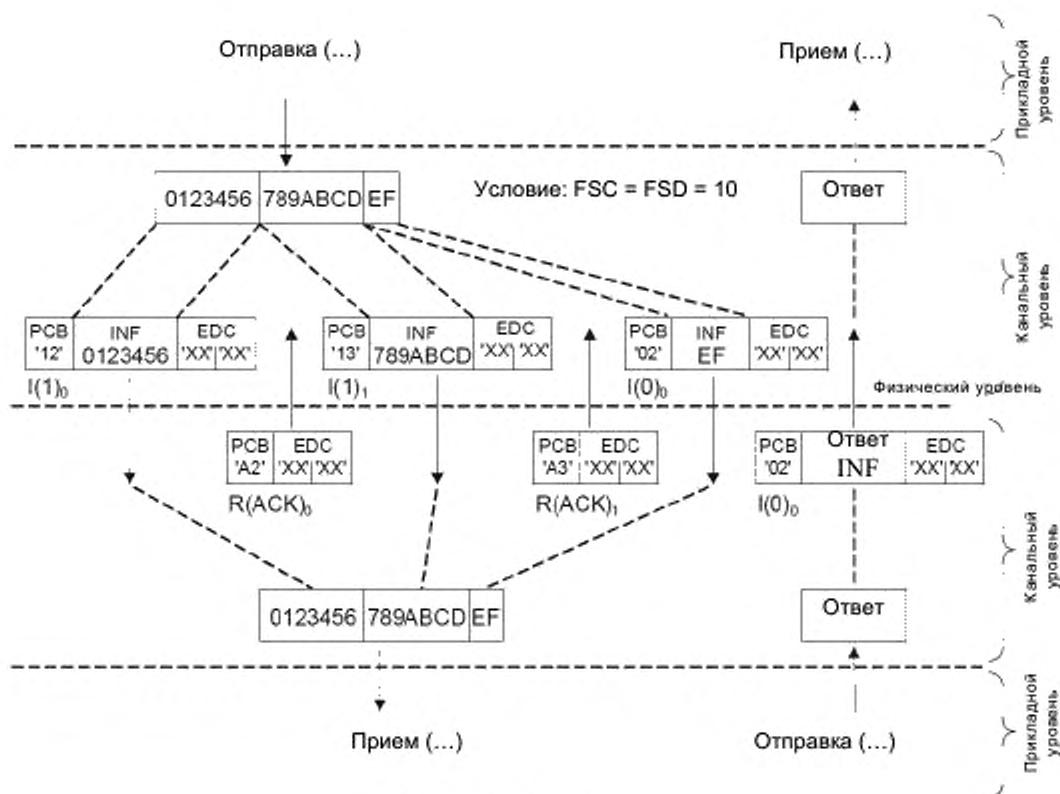
Рисунок 22 – Сцепление
