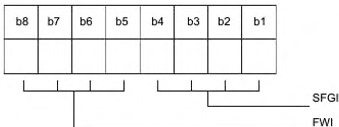
Рисунок 7 – Кодирование байта интерфейса TB(1)
