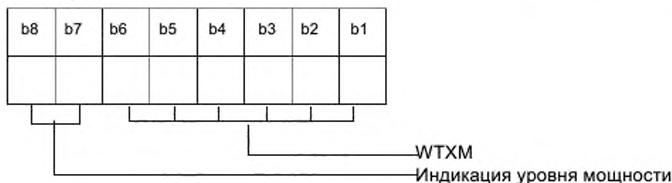
Рисунок 20 – Кодирование INF при запросе S(WTX)
