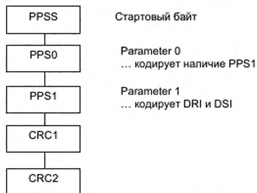
Рисунок 9 – Запрос выбора протокола и параметров
