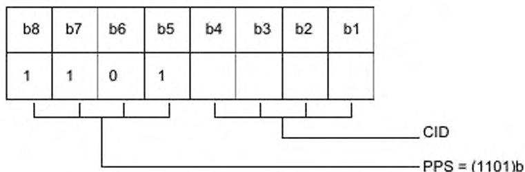
Рисунок 10 – Кодирование PPS
