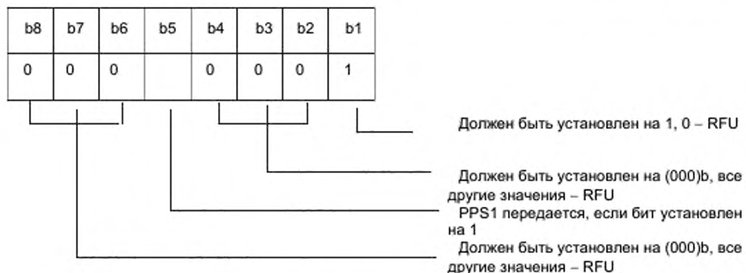
Рисунок 11 – Кодирование PPS0
