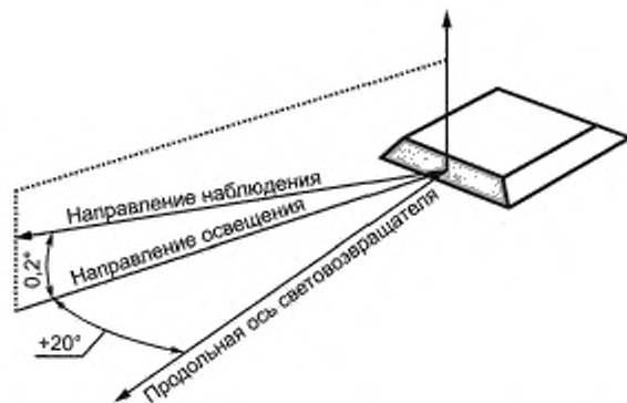
Рисунок 2 — Схема размещения световозвращателя типа КД3 при проведении фотометрических измерений при угле освещения \beta_v = 20^\circ
