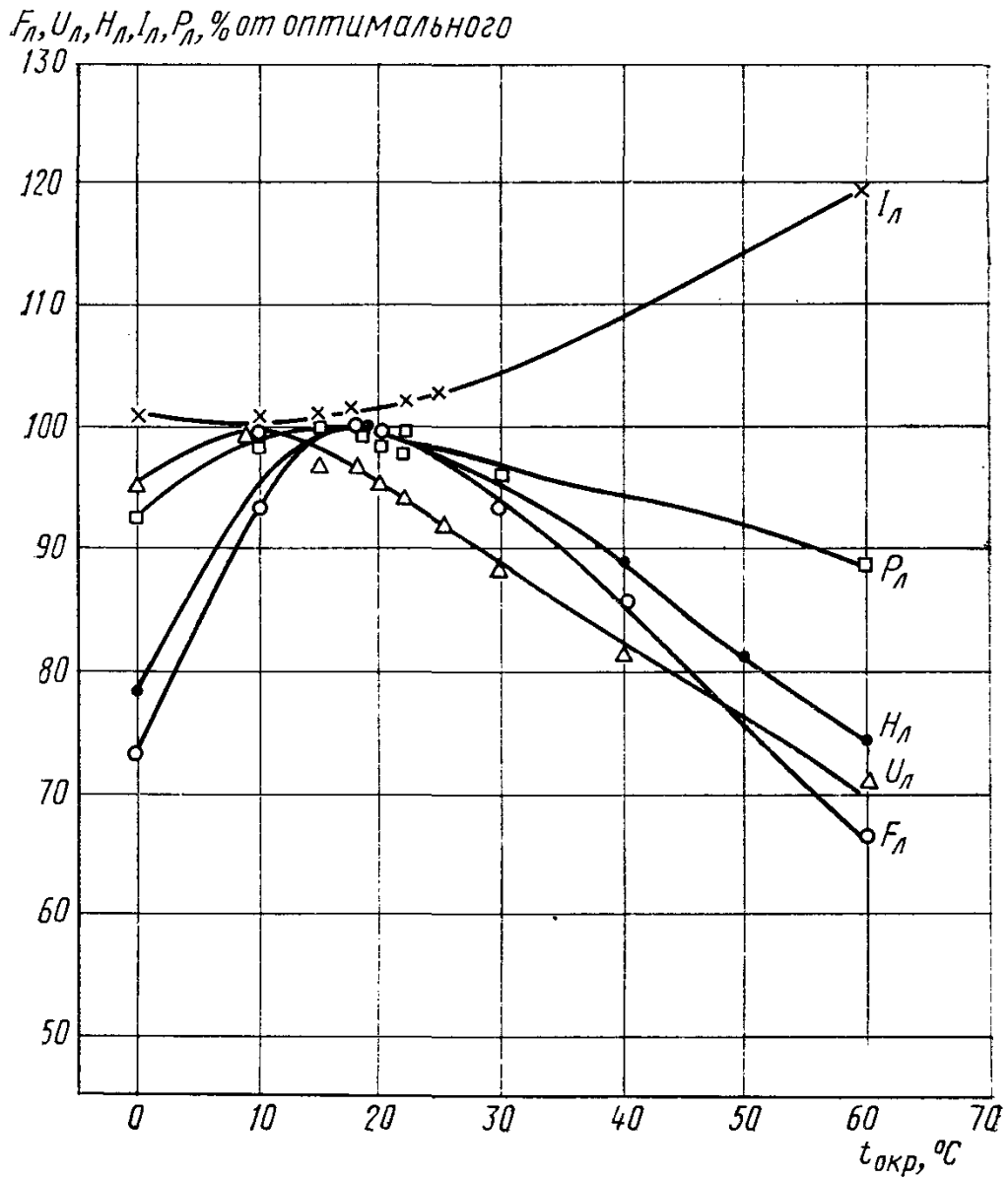
Зависимость параметров люминесцентных ламп мощностью 65 Вт от температуры окружающей среды
