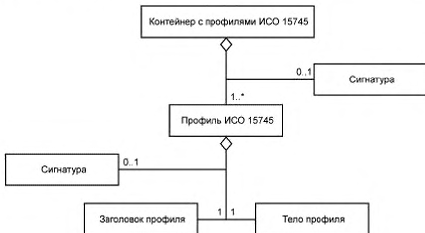
Рисунок 16 — Диаграмма класса контейнера с профилями ИСО 15745
