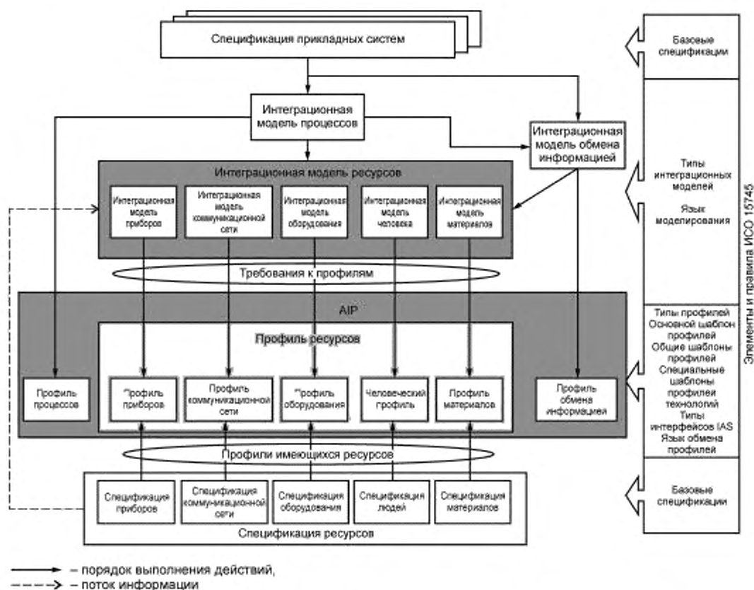
Рисунок 2 — Разработка профилей на основе ИСО 15745
