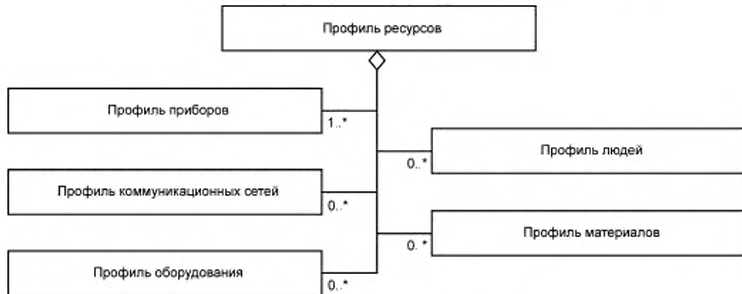
Рисунок 10 — Диаграмма общего класса профиля ресурсов
