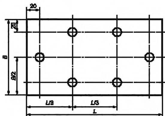
L — длина листа, мм; B — ширина листа, мм
