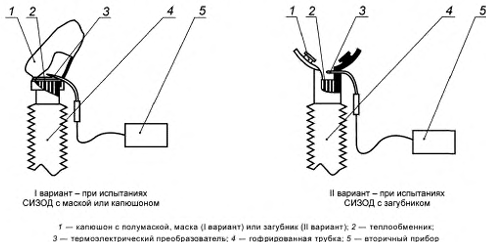
Рисунок 1 — Принципиальная схема измерения температуры вдыхаемой ГДС
