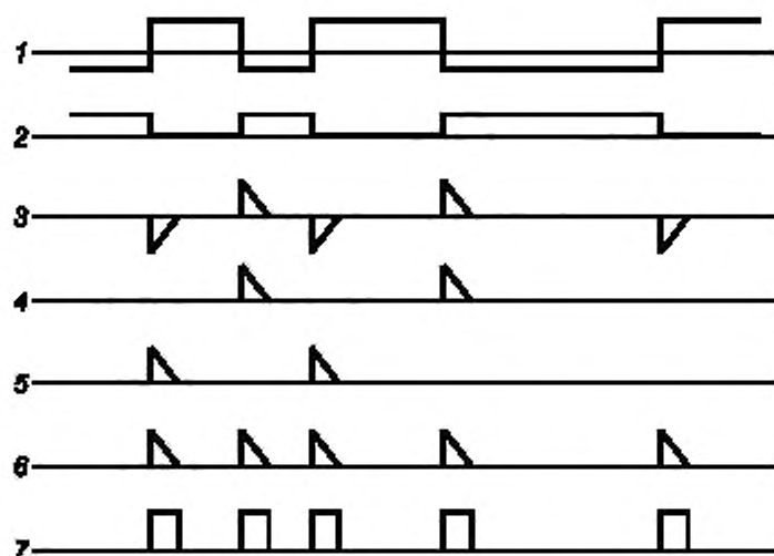
1 — входной сигнал; 2 — сигнал после формирования однополярного сигнала; 3 — сигнал на выходе дифференцирующей цепи; 4 — неинвертируемые положительные импульсы; 5 — сигнал на выходе инвертора; 6 — сигнал на выходе мультивибратора; 7 — выходные импульсы
