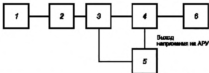
1 — генератор высокочастотных сигналов; 2 — согласующее устройство (эквивалент антенны); 3 — дискретный аттенуатор, 4 — приемник; 5 — осциллограф; 6 — эквивалент нагрузки
