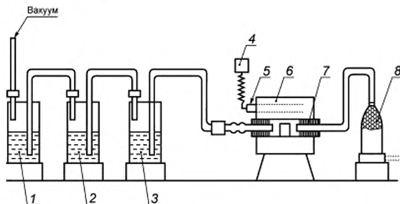
1—3 — склянки Дрекслея поглотительные; 4 — терморегулятор; 5 — термopара; 6 — фарфоровые лодочки; 7 — лодочки фарфоровые; 8 — склянка Тищенко СПТ
