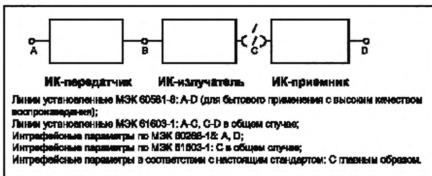
Рисунок 1 — Цепь передачи сигнала и соответствующие стандарты МЭК
