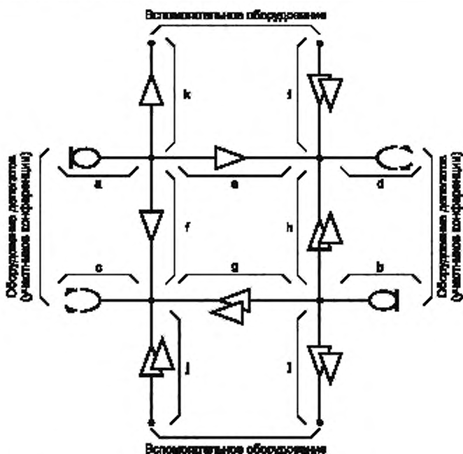
Рисунок 1 — Схемное представление звуковой системы конференц-связи
