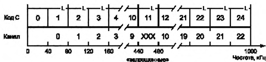
Рисунок 3 — Распределение каналов и рекомендуемые несущие L
