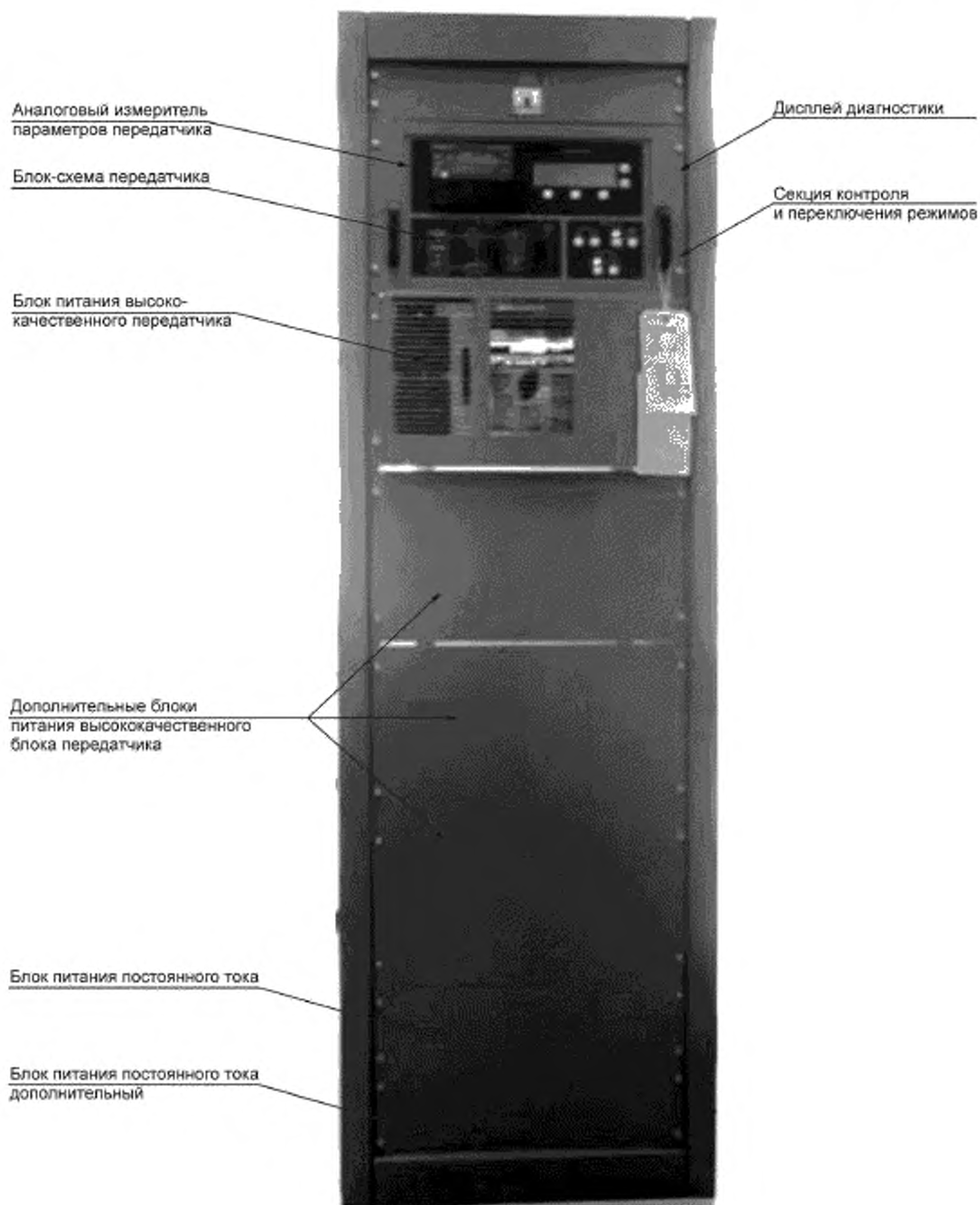
Рисунок 2 — Общий вид радиомаяка «ВЕКТОР D 750»
