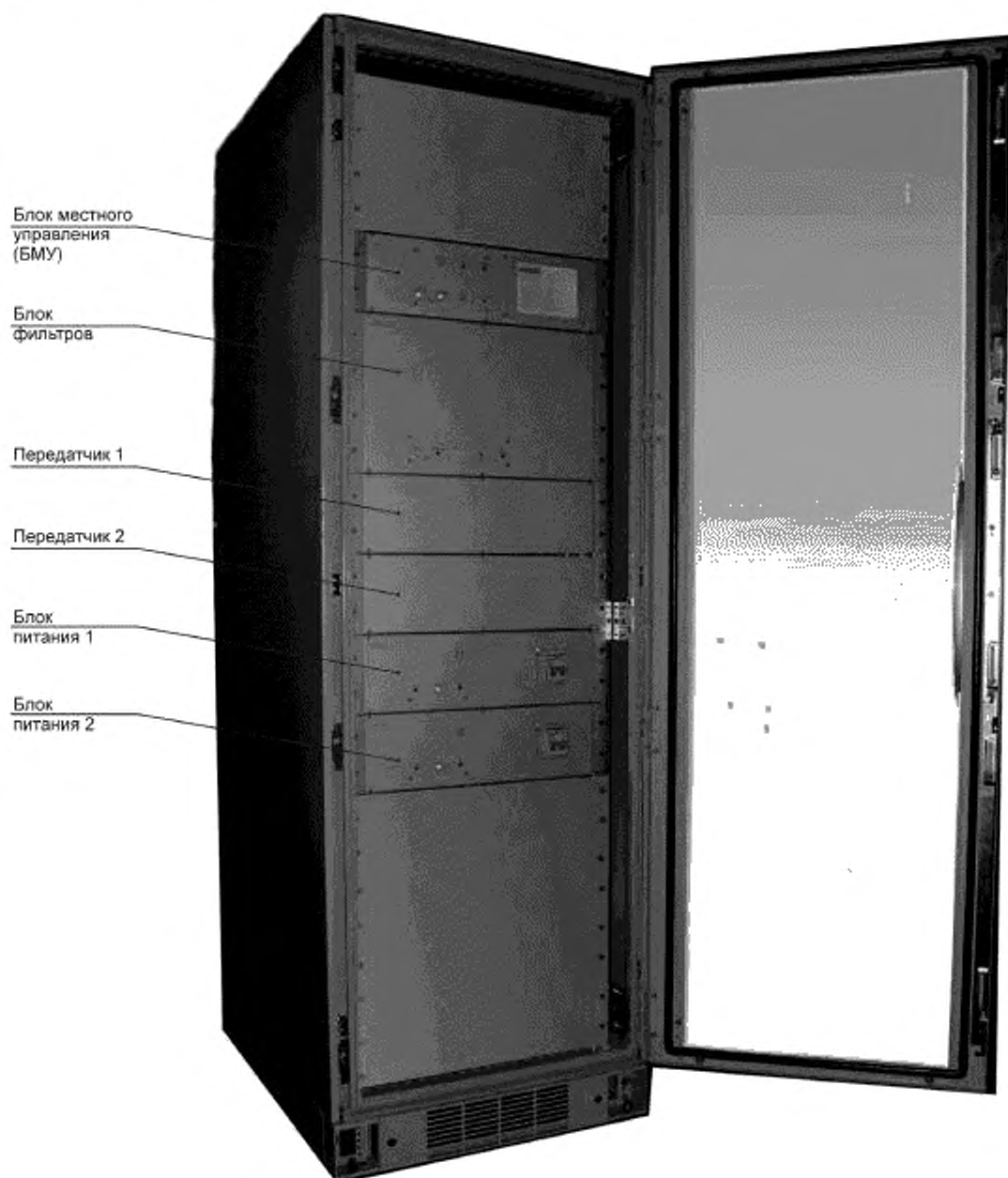
Рисунок 1 — Общий вид радиомаяка «Янтарь-1000»
