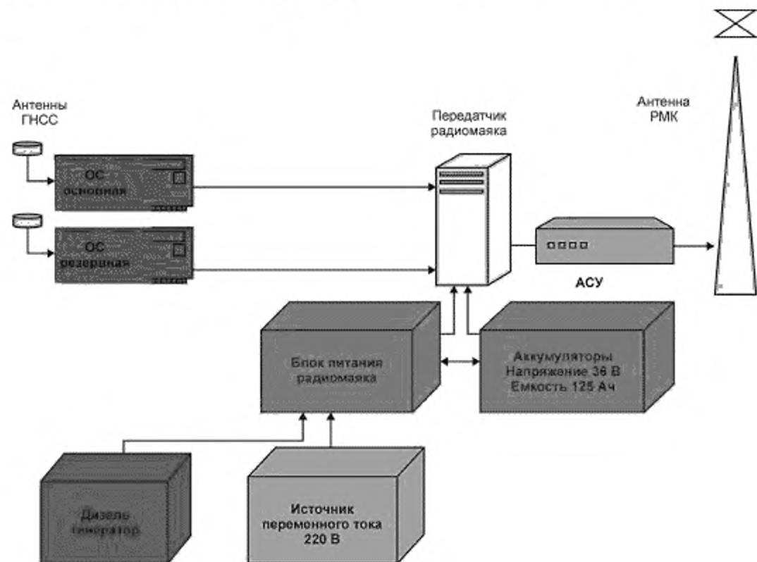
Рисунок 3 — Схема межблочных соединений и питания радиомаяка
