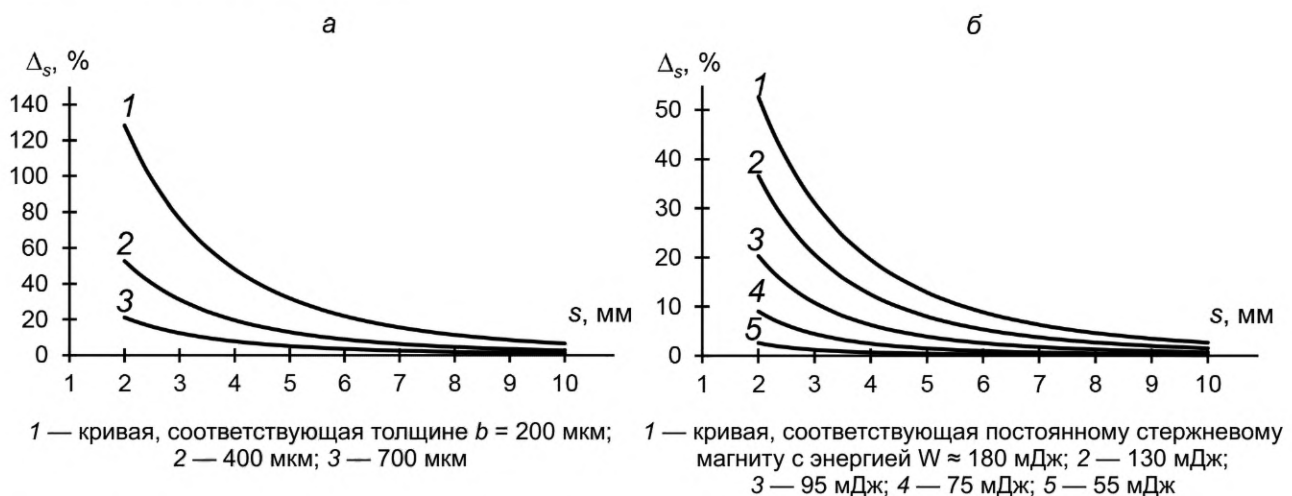
Рисунок 3 — Зависимость дополнительной погрешности \Delta_s , обусловленной намагниченностью корпуса камеры, от толщины s : а — постоянный стержневой магнит с энергией W \approx 180 \text{ мДж} ; б — толщина b = 400 \text{ мкм}
