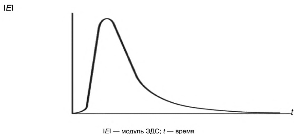
Рисунок 2 — Импульс ЭДС, возникающий в витках катушки магнитодинамического преобразователя при его отрыве и удалении от изделия
