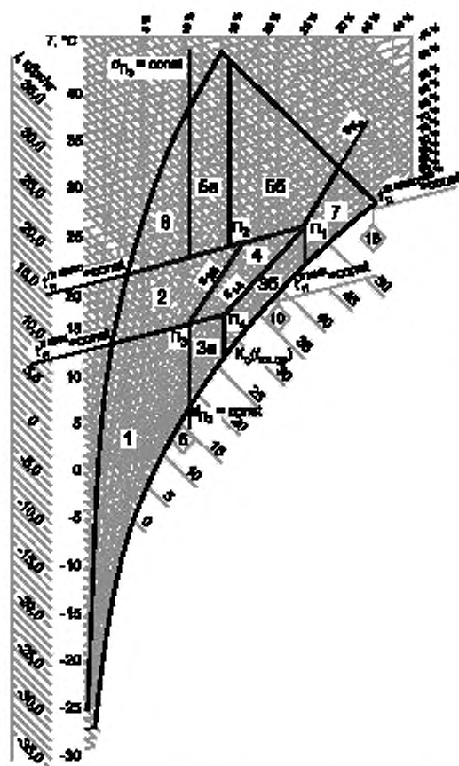
Рисунок 3 — Деление на погодные зоны области возможных сочетаний энтальпии и влагосодержания наружного воздуха для ЦСКВ с пароувлажителем
