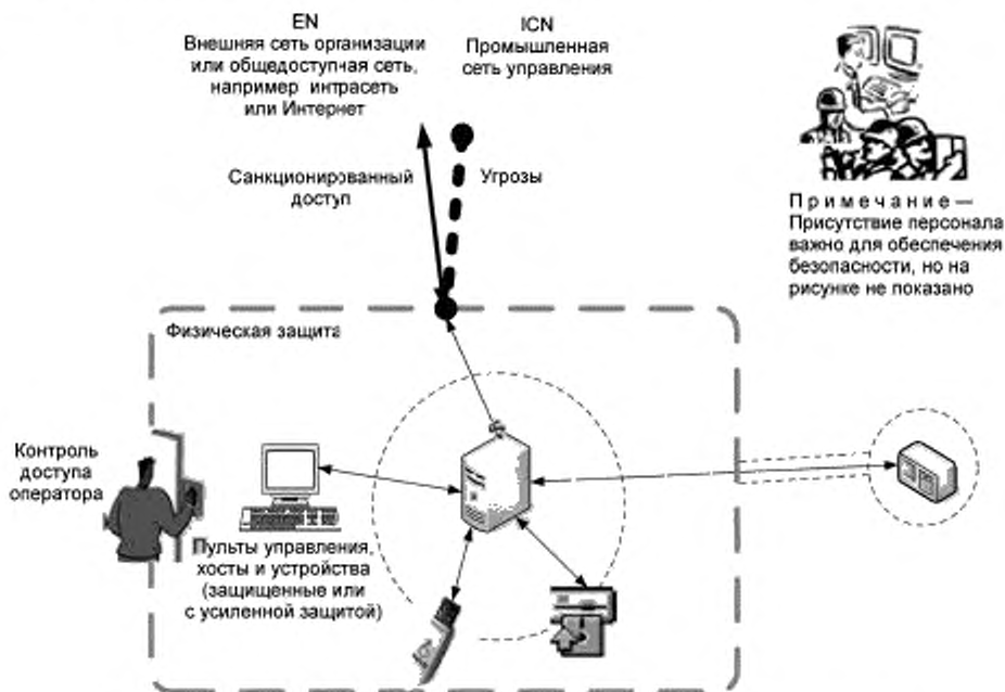
Рисунок 6 — Защита устройства — усиление защиты и управление доступом
