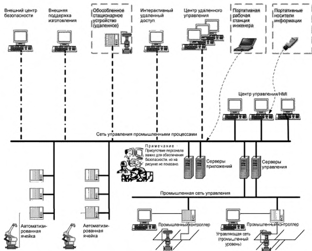
Рисунок 4 — Промышленная система управления (ICS)
