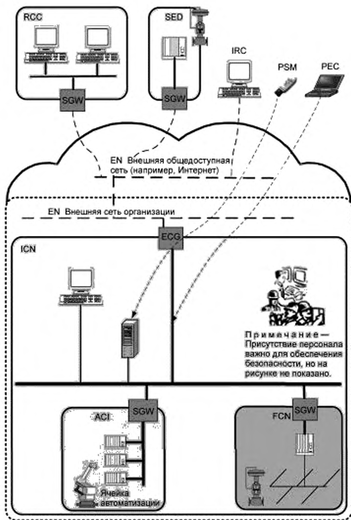
Рисунок 8 — Пример — сегментация ICS
