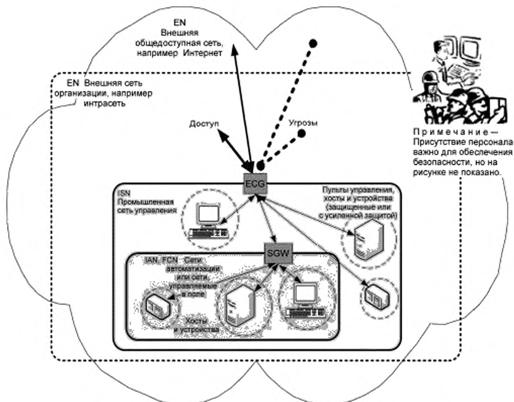
Рисунок 7 — Эшелонированная оборона за счет использования сегментации
