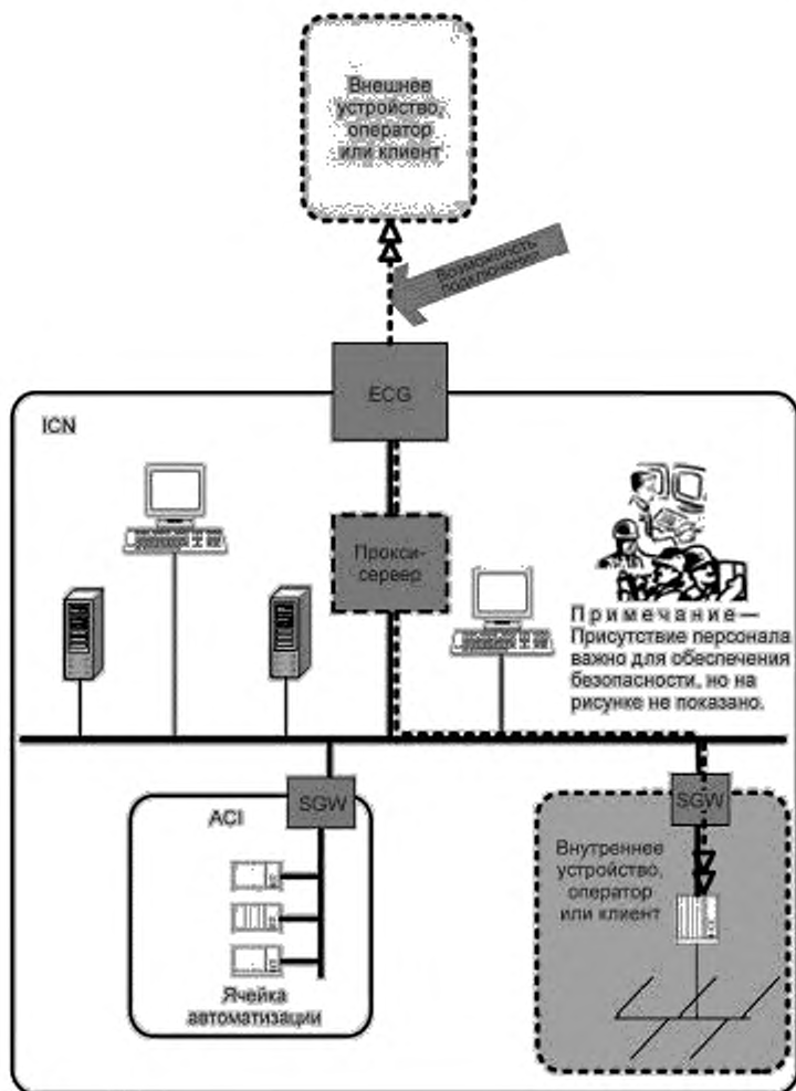
Рисунок 9 — Общие внешние соединения
