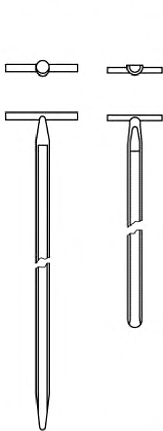
Рисунок 2 — Совковые пробоотборники для взятия проб порошков
