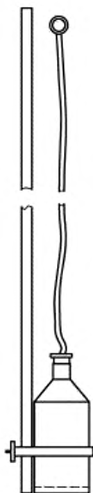
Рисунок 6 — Бутыль для отбора проб
