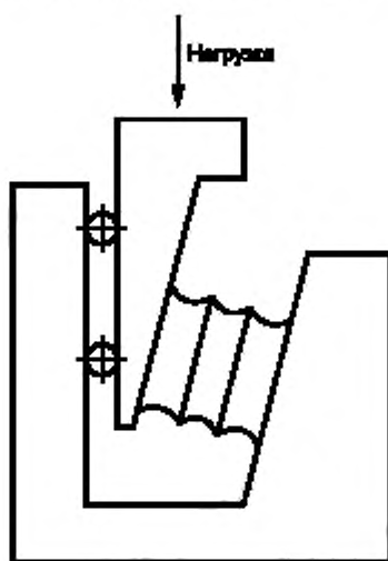
Рисунок 2 — Установка рессоры на стенде
