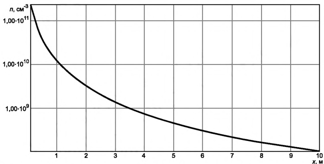
Рисунок Б.2 — Распределение концентрации плазмы n , \text{см}^{-3} , в струе двигателя СПД-100 вдоль оси струи (логарифмическая шкала)
