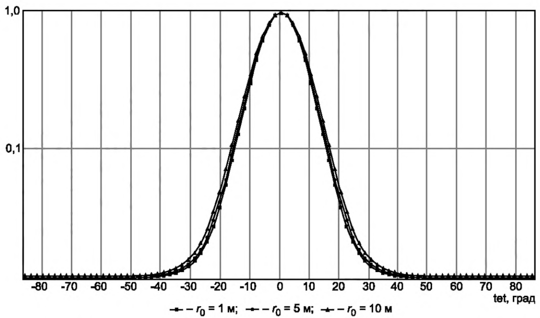
Рисунок Б.6 — Распределение энергии ионов E/E_c поперек струи для двигателя СПД-100
