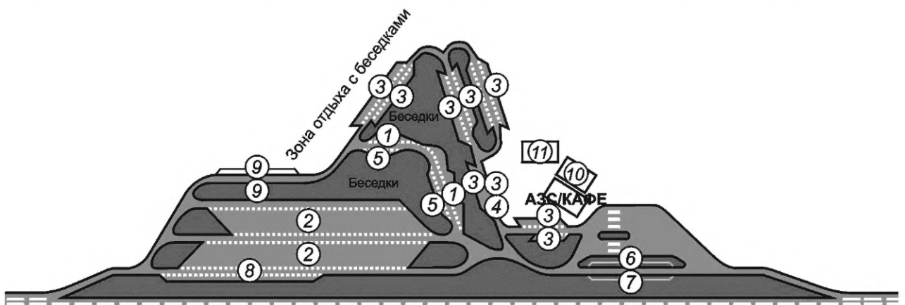
Рисунок А.2 — Вариант 2 размещения автозаправочной станции совместно с кафе и площадкой отдыха
