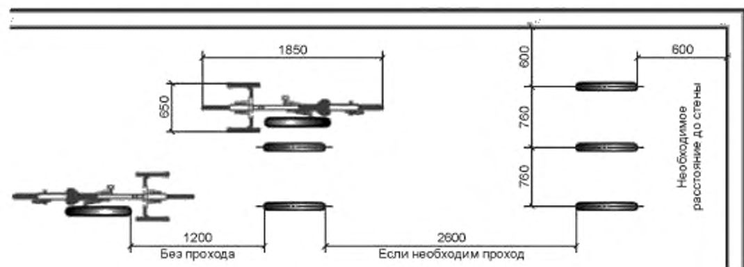
Рисунок 1 — Минимальные необходимые расстояния для создания велопарковки
