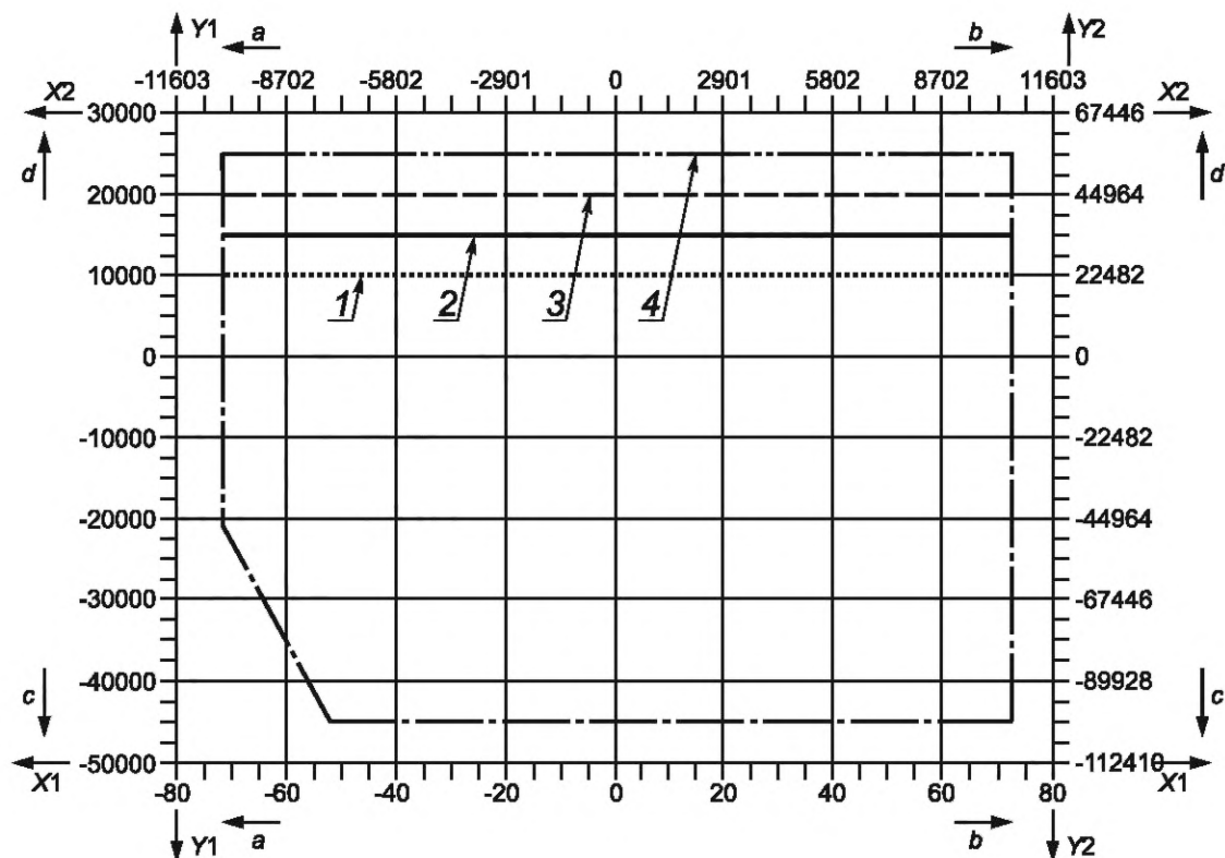
X1 — давление, МПа; X2 — давление, фунт/дюйм 2 ; Y1 — сила, даН; Y2 — сила, фунт; 1 — область для 10 000 даН (212 482 фунт) срез. кольцо; 2 — область для 15 000 даН (33 723 фунт) срез. кольцо; 3 — область для 20 000 даН (44 964 фунт) срез. кольцо; 4 — область для 25 000 даН (956 205 фунт) срез. кольца; a — выше; b — ниже; c — сжатие; d — растяжение
