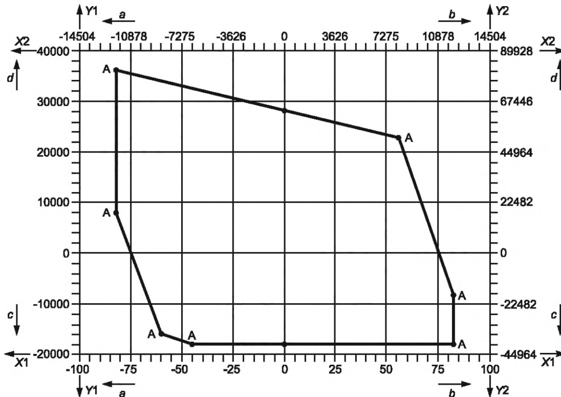
Рисунок 1 — Пример номинальных значений рабочих характеристик
