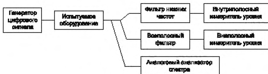
Рисунок 6 — Схема соединения оборудования
