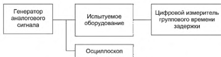
Рисунок 19 — Схема соединения оборудования
