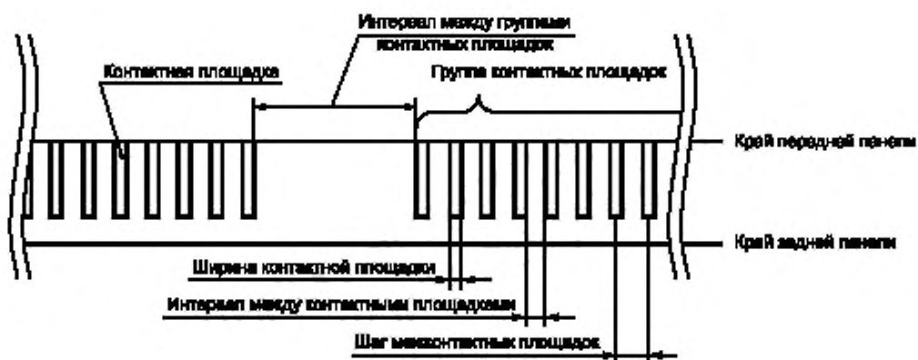
Рисунок Е.2 — Размеры контактных площадок
