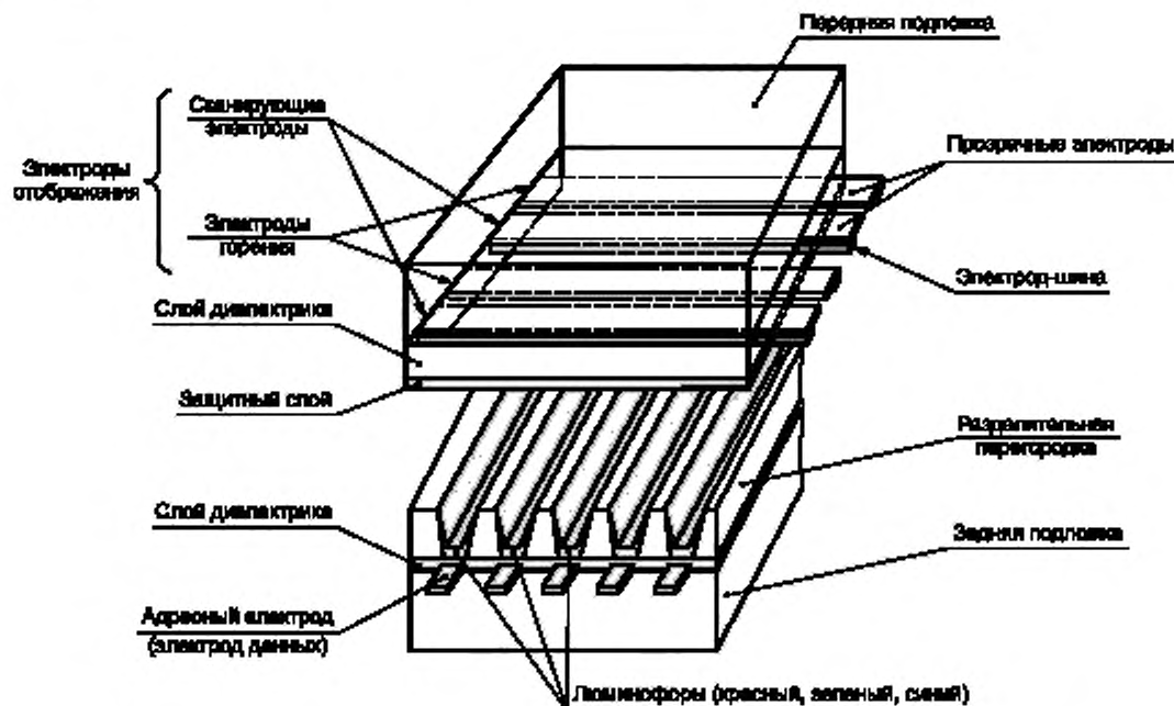
Рисунок А.7 — Структура цветной AC PDP трехэлектродного типа и поверхностным разрядом
