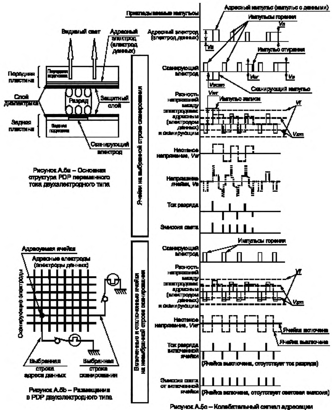
Рисунок А.5 — Работа AC PDP двухэлектродного типа
