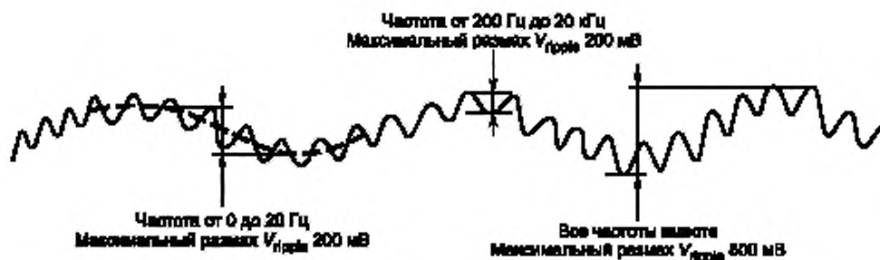
Рисунок 2 — Максимальное напряжение пульсаций (размах)
