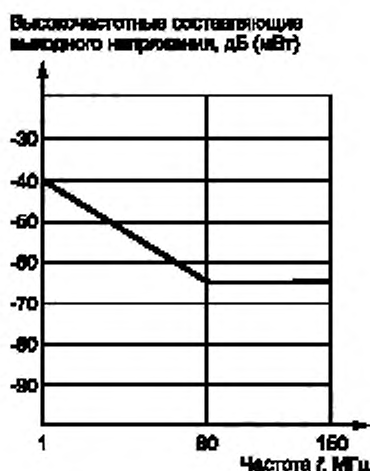
Рисунок 3 — Максимальные ВЧ составляющие выходного напряжения
