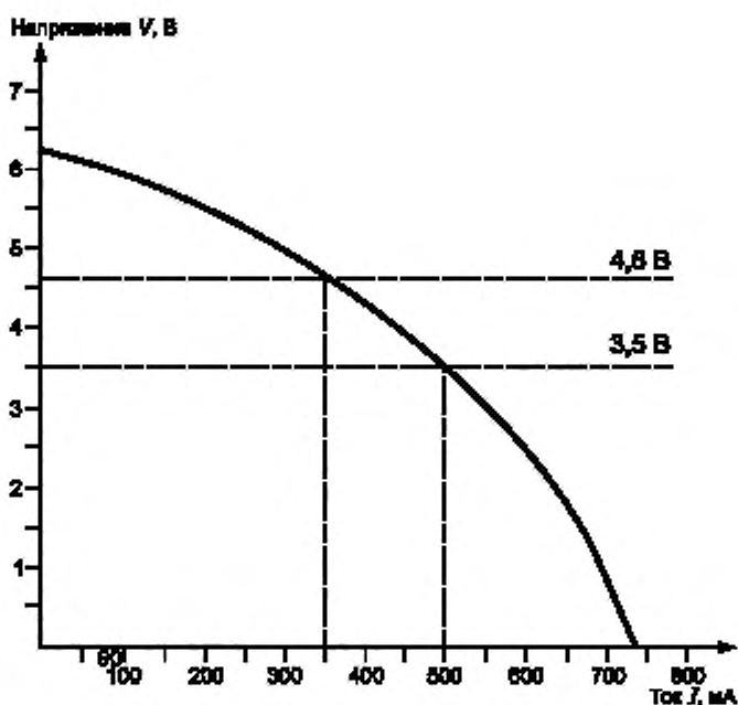
Рисунок 7 — Требования к линейности тока
