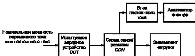
Рисунок 4 — Испытательная установка для проверки ВЧ составляющих напряжения
