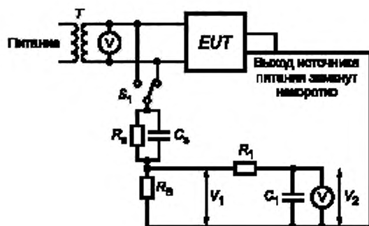
Рисунок 5 — Испытательная установка
