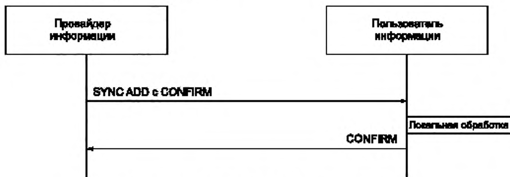
Рисунок А.6 — Транзакция SYNC ADD с подтверждением
