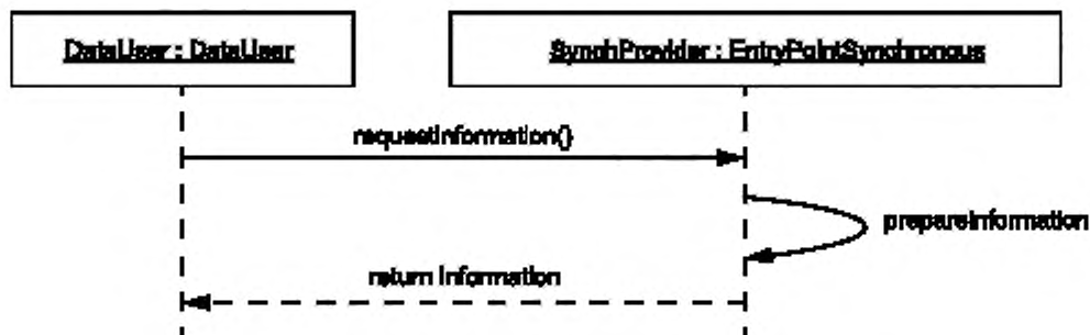
Рисунок 4 — Пример применения синхронного интерфейса «запрос-ответ»
