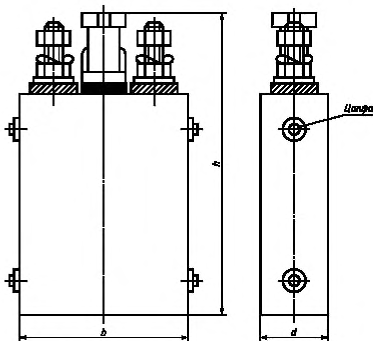
Рисунок 1 — Пример призматического аккумулятора
