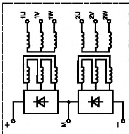
Рисунок 5а — Трехфазное электрооборудование с двумя группами элементов
