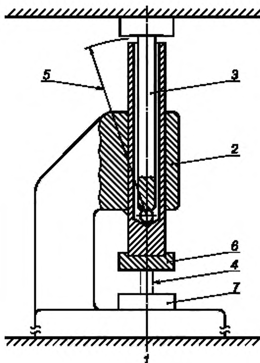
1 — машина для испытания; 2 — направляющая рама; 3 — пуансон; 4 — образец; 5 — радиус; 6, 7 — плита
