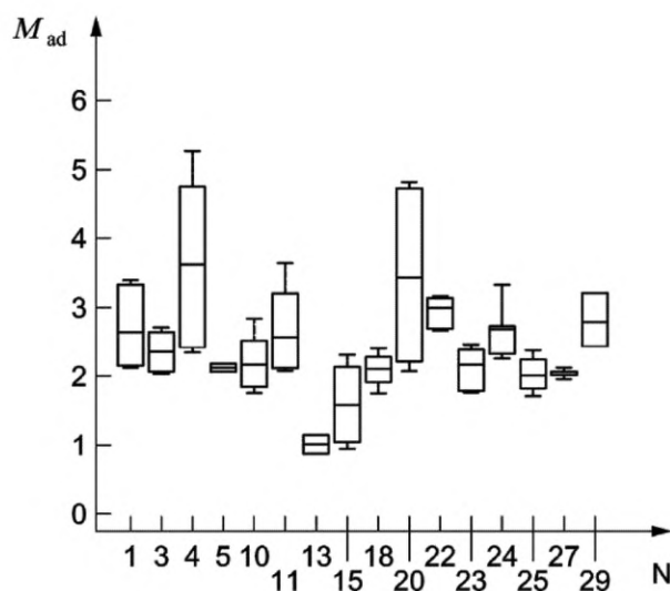
Рисунок А.1 — Отклонение результатов испытаний между лабораториями. Измельченные шины
