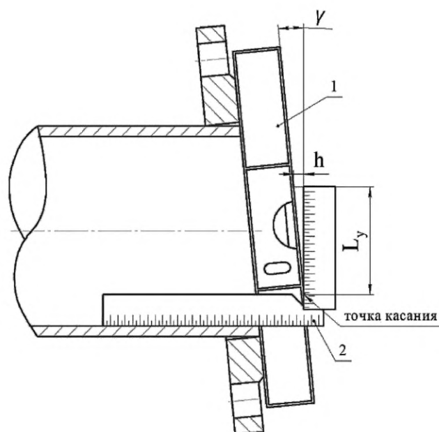
1 — уровень, 2 — угольник
