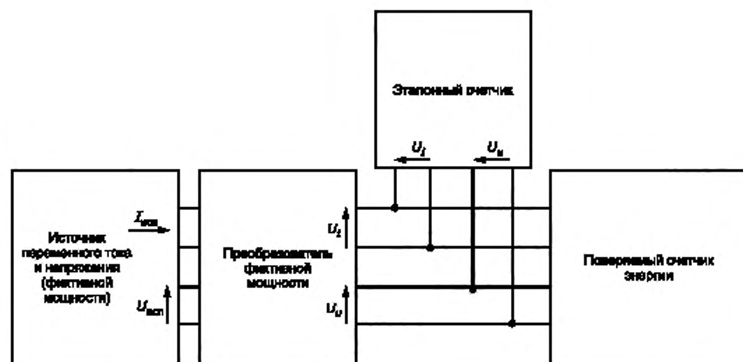
Рисунок А.2 — Схема испытательной цепи с применением источника и преобразователя фiktивной мощности, эталонного ЭлТА-счетчика с входами « U_I » и « U_U » для проверки однофазного ЭлТА-счетчика
