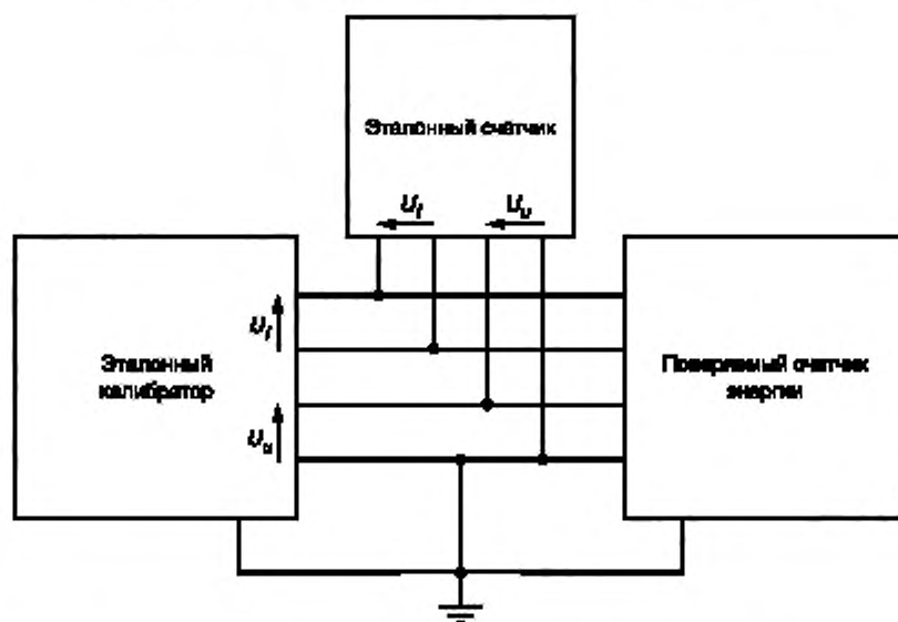
Рисунок А.1 — Схема испытательной цепи с применением калибратора для проверки однофазного ЭлТА-счетчика
