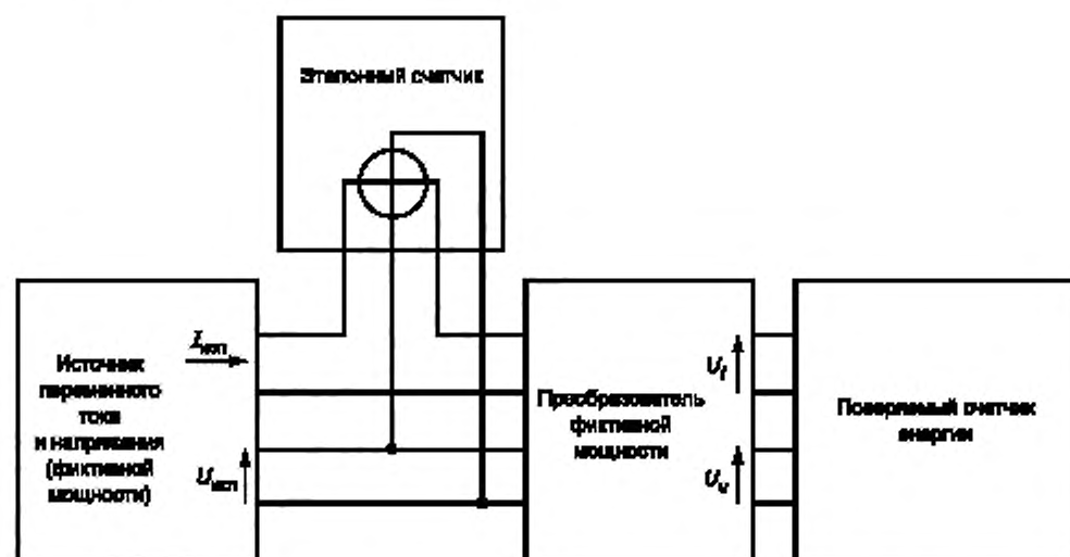
Рисунок А.3 — Схема испытательной цепи с применением источника и преобразователя фиктивной мощности, эталонного ЭЛТА-счетчика с входами «U» и «I» для проверки однофазного ЭЛТА-счетчика
