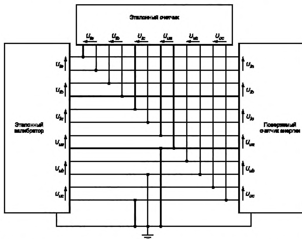
Рисунок А.4 — Схема испытательной цепи с применением калибратора для проверки трехфазного ЭЛТА-счетчика
