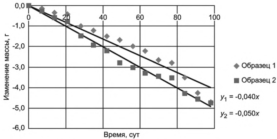
Рисунок А.3 — Абсолютное изменение массы образцов ОПТИМА в процессе испытаний
