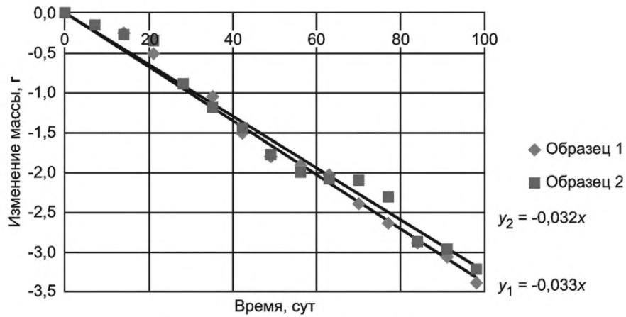
Рисунок А.2 — Абсолютное изменение массы образцов СТАНДАРТ в процессе испытаний
