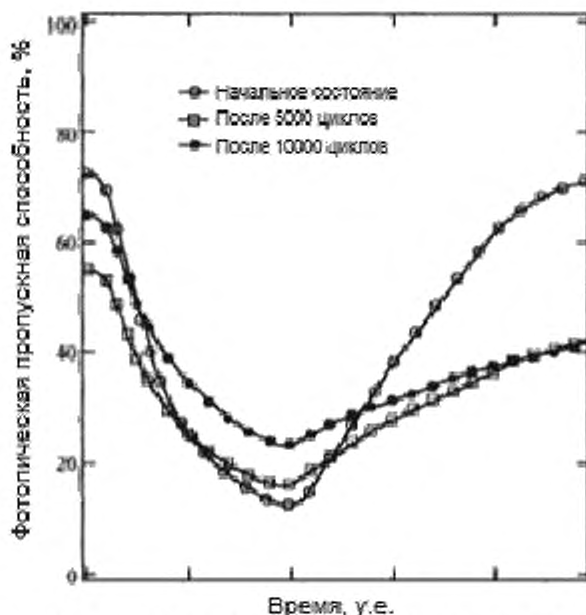
Рисунок 5 — Фотопропускная способность как функция времени, измеренного на различных этапах циклических испытаний типичного ЭХП стеклопакетов
