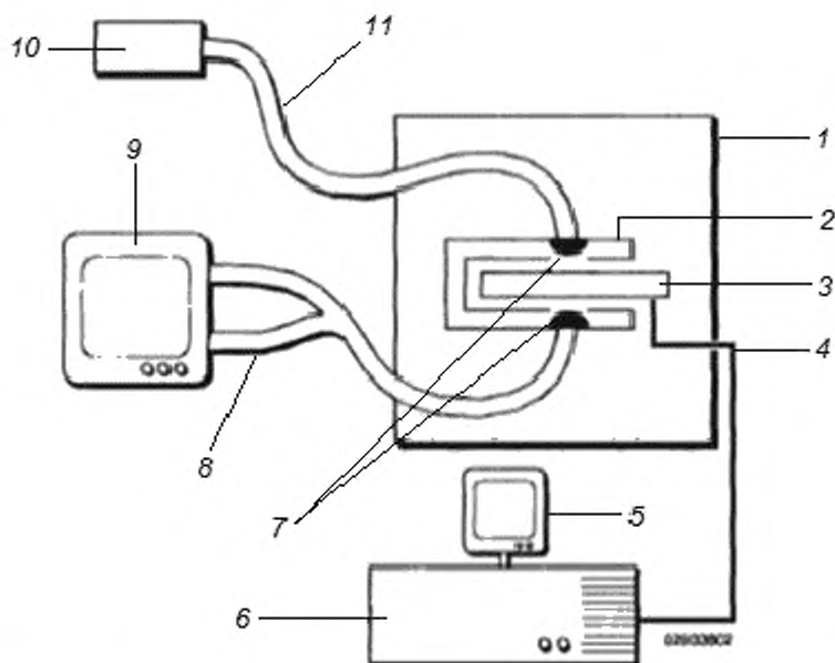
1 — конвекционная печь; 2 — держатель образца; 3 — электрохромное окно; 4 — электрические выводы и камеры термодар; 5 — компьютер; 6 — многоканальная цифровая автоматизированная система управления и сбора данных; 7 — коллимирующая линза; 8 — оптоволоконный кабель-разветвитель; 9 — вычислитель спектрофотометра с фотодиодной матрицей; 10 — лампа накаливания; 11 — оптоволоконный кабель
