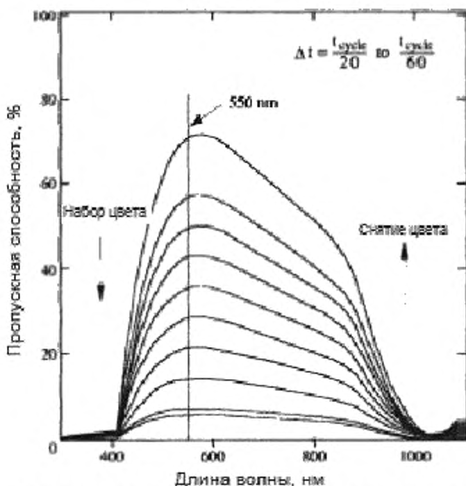
Рисунок 4 — Спектры пропускания в течение набора цвета и снятия цвета при интервалах в диапазоне от t_{\text{cycle}}/20 до t_{\text{cycle}}/60 у типовых ЭХП стеклопакетов
