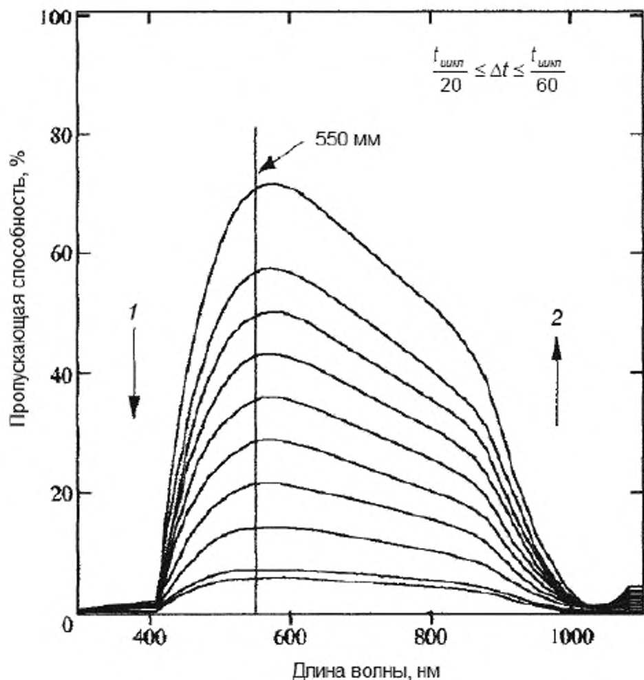
1 — состояние с установленным цветом; 2 — бесцветное состояние
