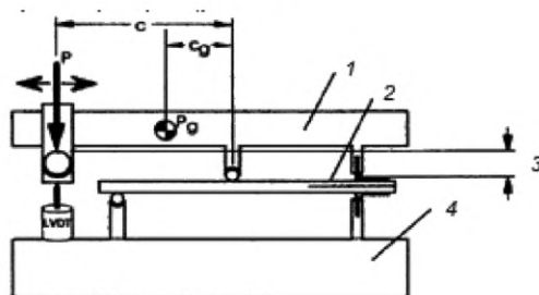
1 — рычаг; 2 — образец испытаний; 3 — погрузочная высота; 4 — основание
