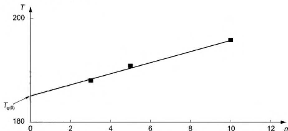
Рисунок 2 — Определение T_{g(0)} при 0 °C/мин по калибровочному графику
