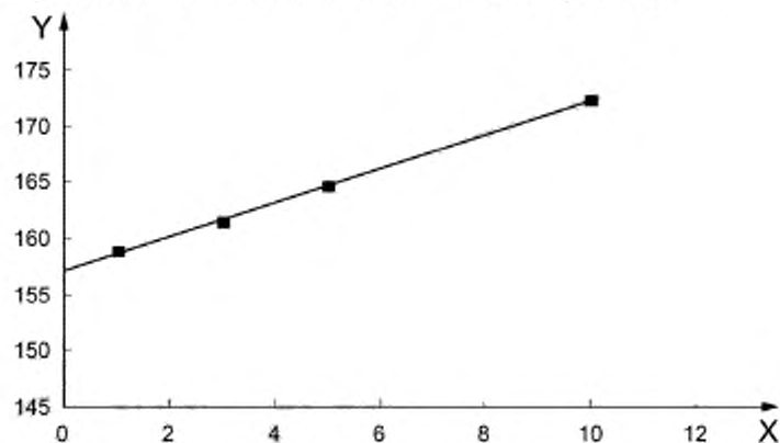
Рисунок А.2 — График зависимости кажущейся температуры плавления индия (определенной по графику модуля потерь) от скорости нагревания
