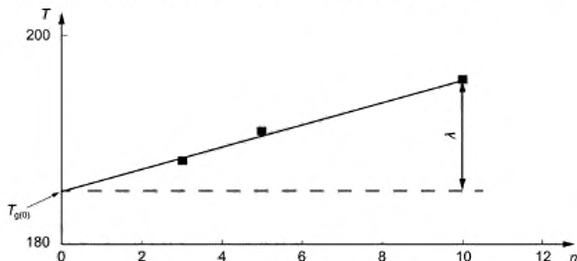
Рисунок 3 — Определение T_{g(n)} для заданной скорости нагревания по калибровочному графику
