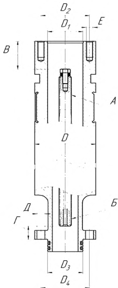
Рисунок К.1 — Габаритные и присоединительные размеры гидрозакщит с диаметром корпуса 69; 81; 86; 92; 103; 114 мм
