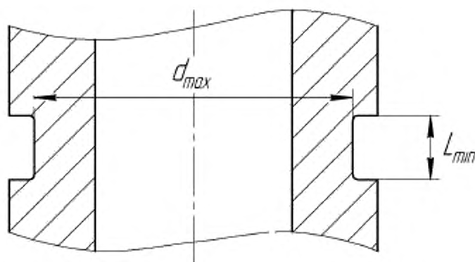
Рисунок И.2 — Размеры посадочного места для хомутов-звездаторов на электродвигатели с диаметром корпуса 81; 96; 103; 117; 130 мм
