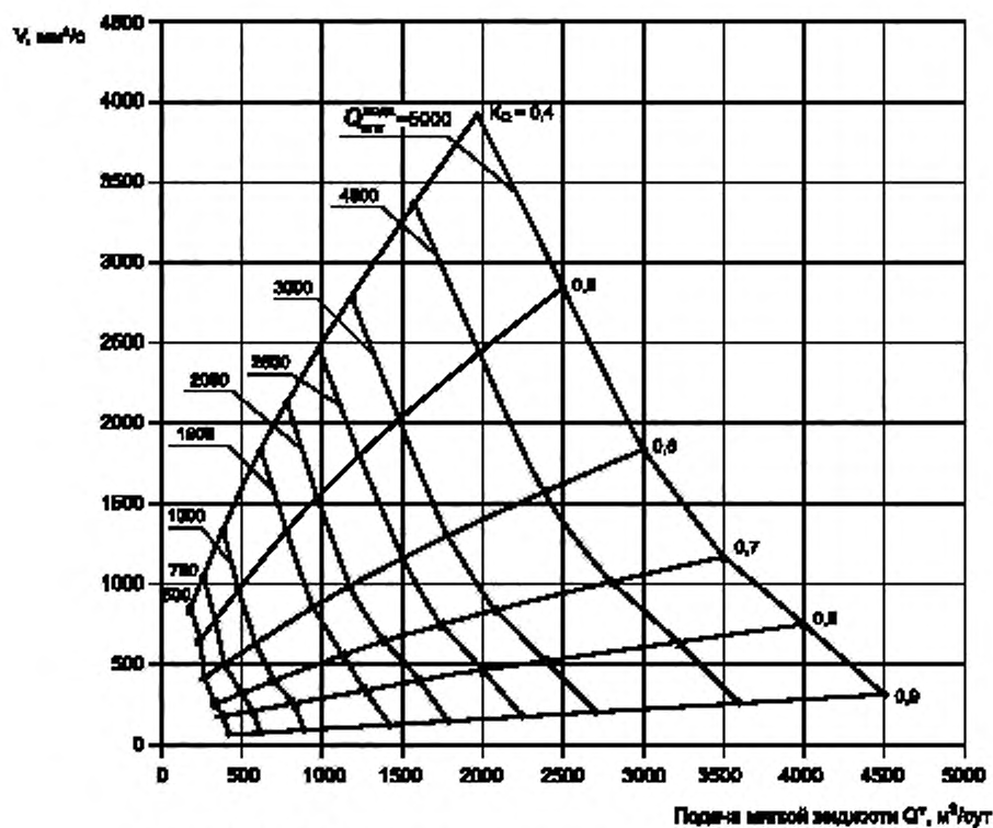
Рисунок А.1 — График изменения оптимальной подачи центробежного и диагонального насоса ( Q_{\text{опт}}^{\text{вода}} = 500 - 5000 \text{ м}^3/\text{сут} )
