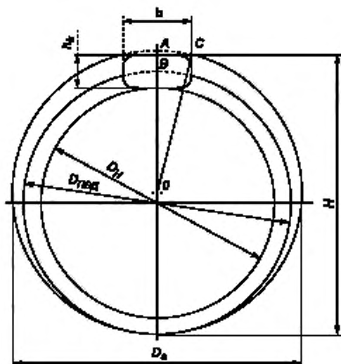
Рисунок 1 — Сечение погружной части УЭЛН, без защитного устройства плоского кабеля
