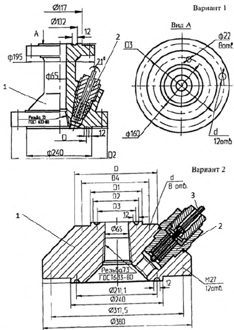
Рисунок 6 — Схема уплотнительного устройства кабельной линии УЭЛН при низком затрубном давлении (до 7,0 МПа)
