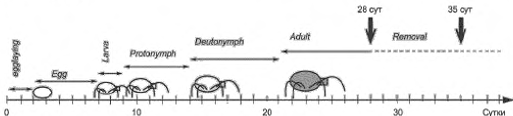
Рисунок С.1 — Развитие Hypoaspis (Geolaelaps) aculeifer при температуре 20 °С
