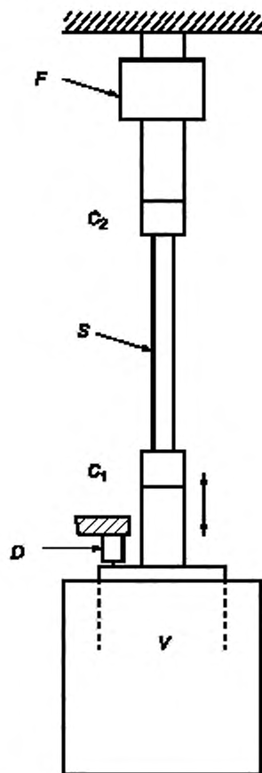
F — датчик силы; C_1 , C_2 — зажимы; S — образец для испытания; D — датчик смещения; V — вибратор
