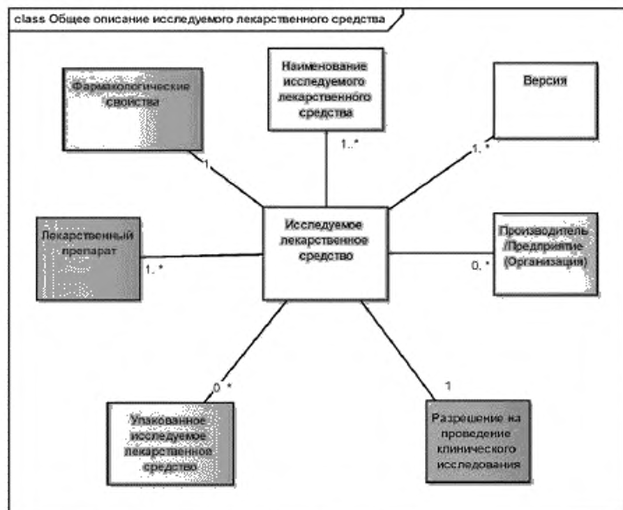
Рисунок 21 — Общая модель информации об исследуемом лекарственном средстве
