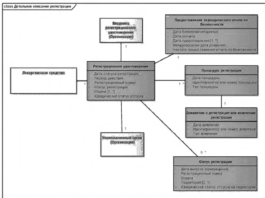
Рисунок 9 — Детальная модель информации о регистрации
