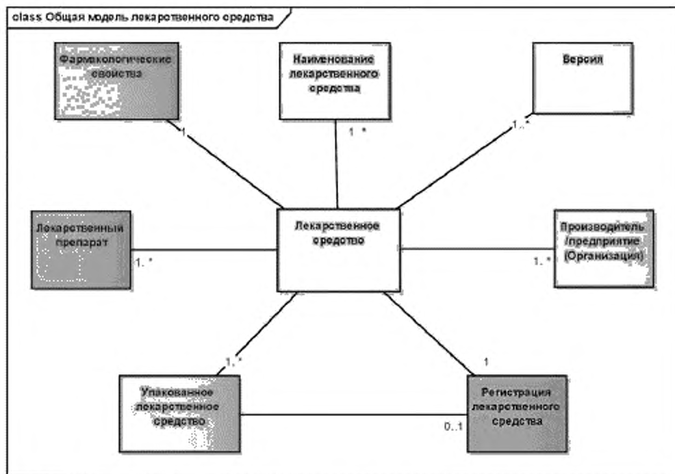
Рисунок 5 — Общая модель информации о лекарственном средстве
