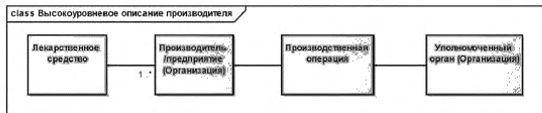
Рисунок 11 — Высокоуровневая модель информации о производителе или предприятии
