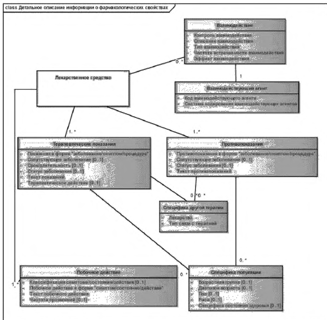
Рисунок 20 — Детальное описание информации о фармакологических свойствах
