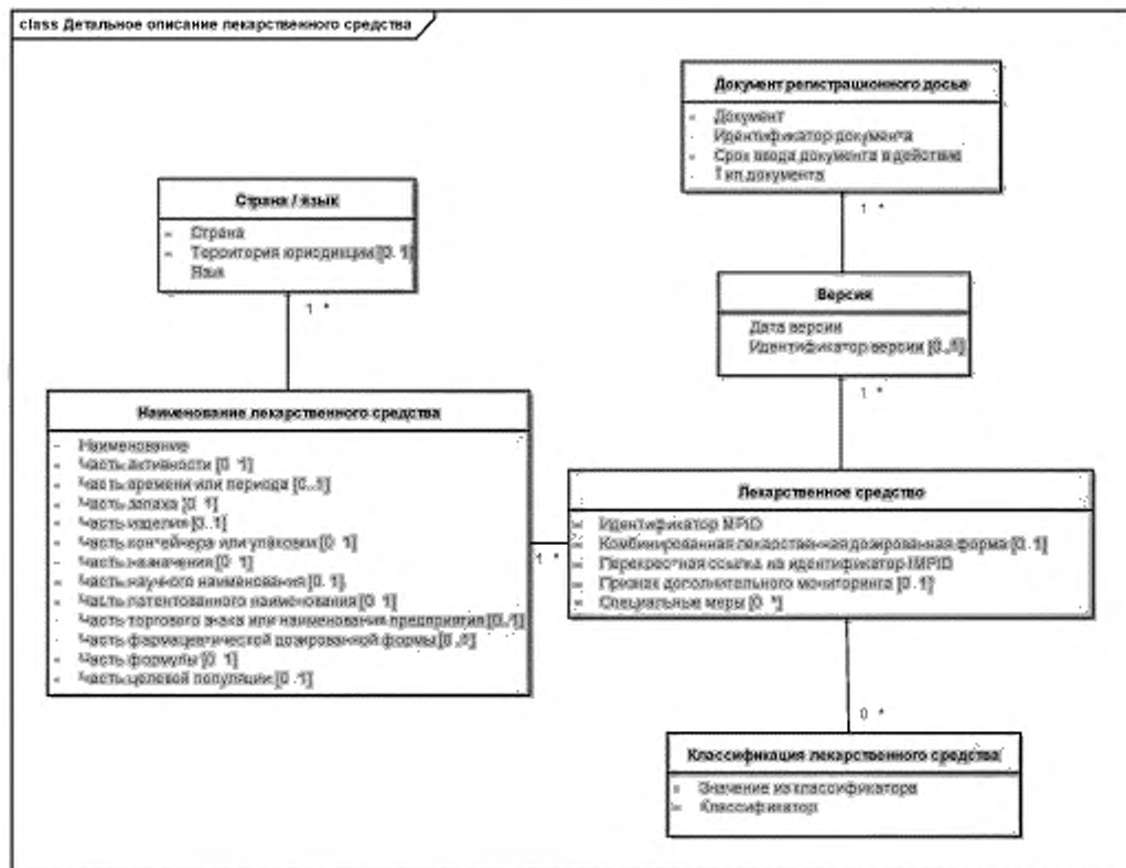
Рисунок 7 — Детальная диаграмма описания раздела лекарственного средства
