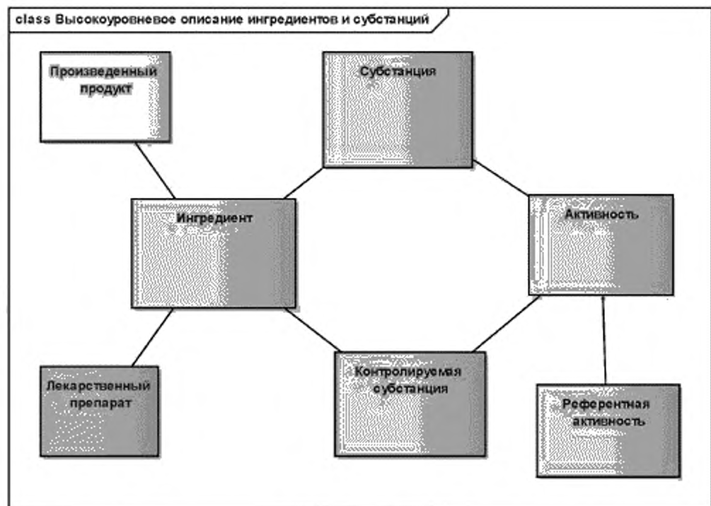
Рисунок 15 — Высокоуровневое описание раздела ингредиента, субстанции и активности
