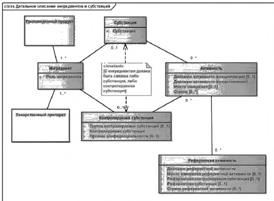
Рисунок 16 — Детальное описание раздела ингредиента, субстанции и активности
