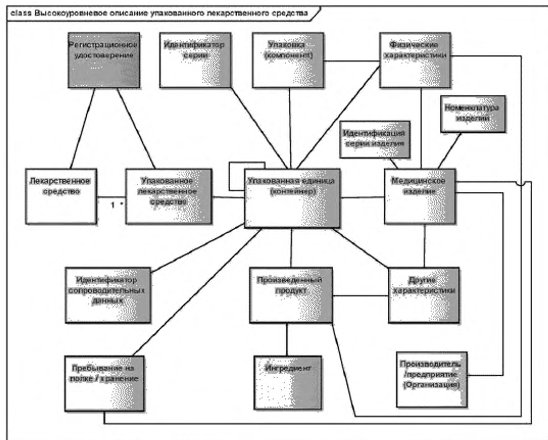
Рисунок 13 — Высокоуровневое описание раздела упакованного лекарственного средства
