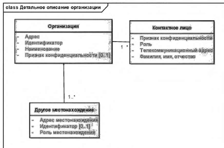
Рисунок 10 — Детальная модель информации об организации
