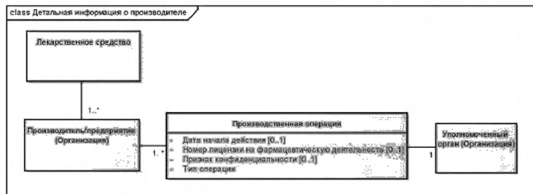
Рисунок 12 — Детальная модель информации о производителе или предприятии
