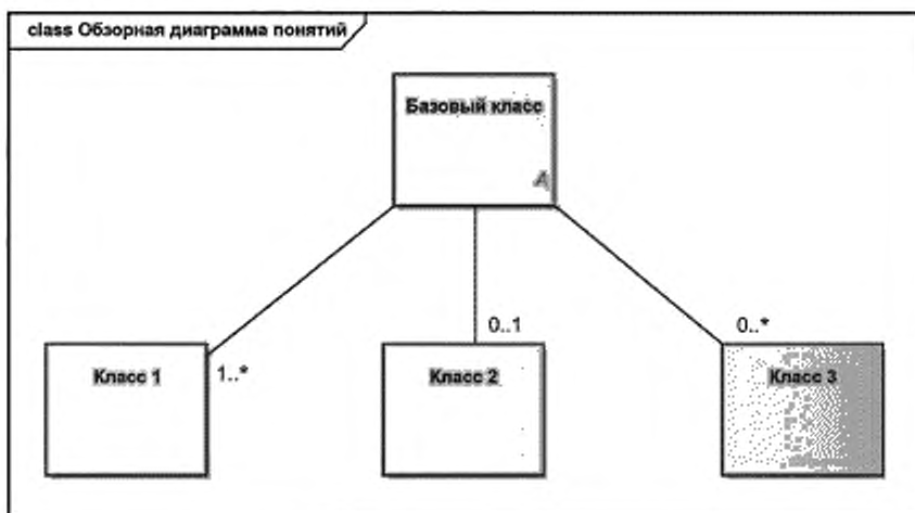
Рисунок 2 — Пример концептуальной обзорной диаграммы
