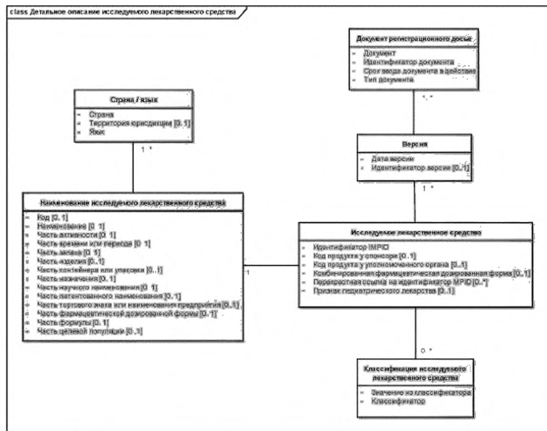
Рисунок 22 — Детальное описание раздела исследуемого лекарственного средства
