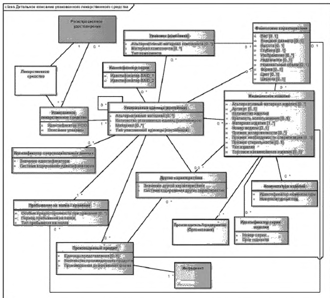
Рисунок 14 — Детальное описание информации об упакованном лекарственном средстве
