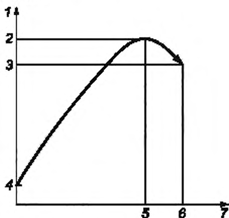
Рисунок 1 — Пример кривой зависимости «усилие — относительное удлинение»
