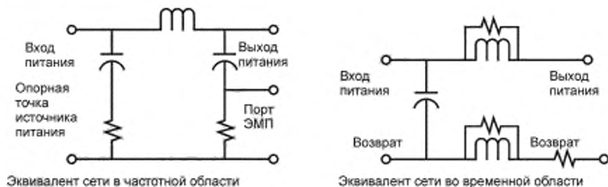
Рисунок Г.1 — Схемы эквивалентов сети
