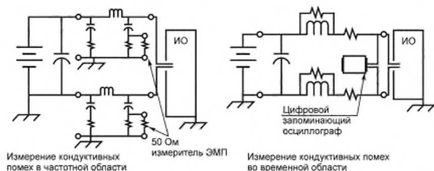
Рисунок Г.2 — Моделирование кондуктивных помех в частотной и временной областях
